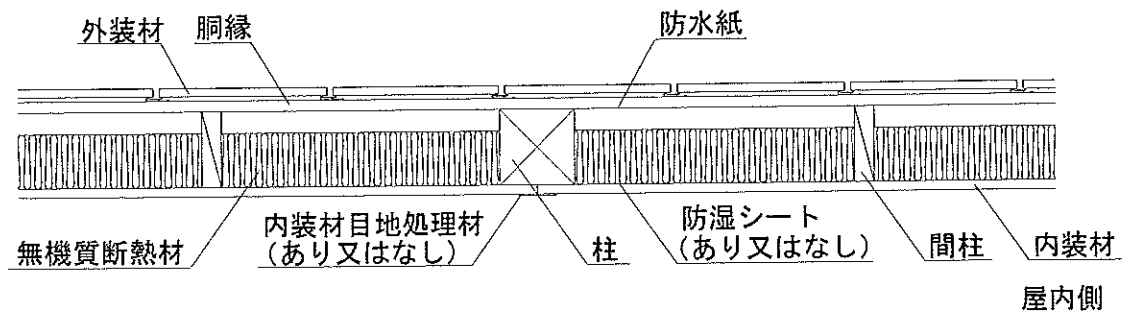
水平断面図
