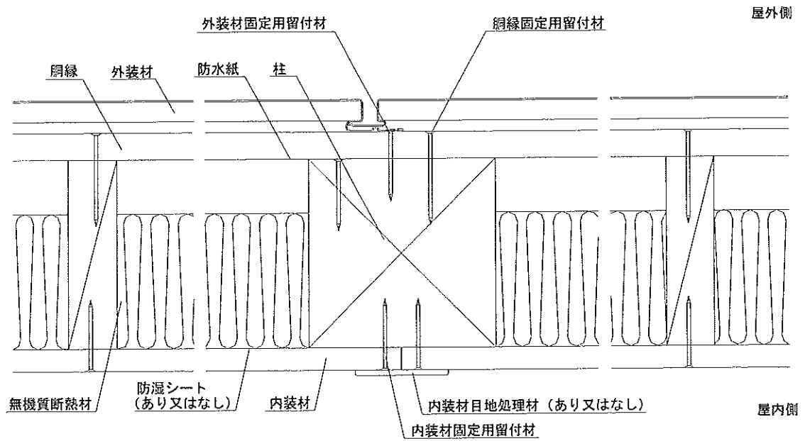
水平断面図
