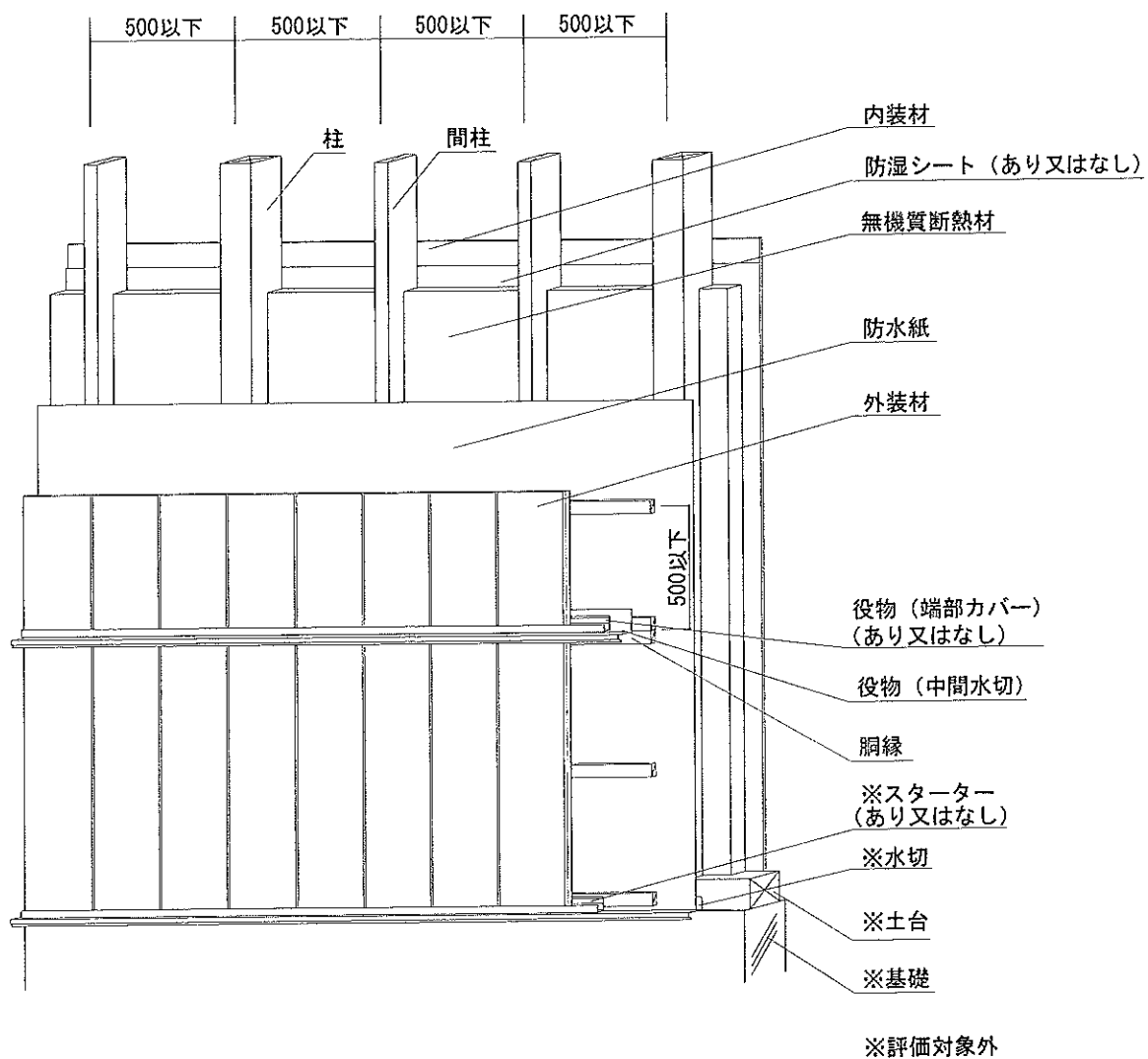
透視図
