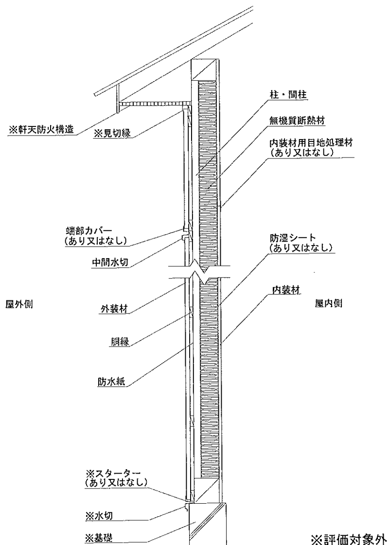
鉛直断面図
