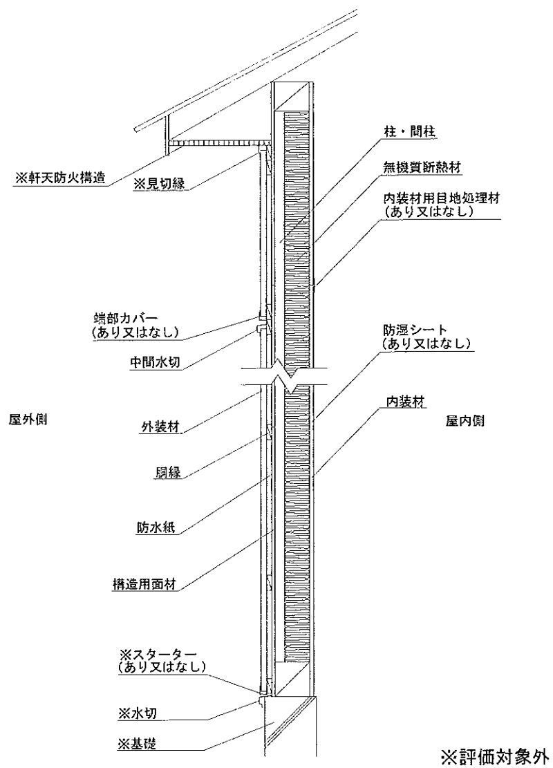
鉛直断面図
