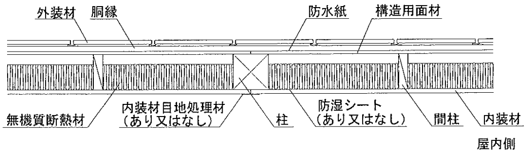
水平断面図
