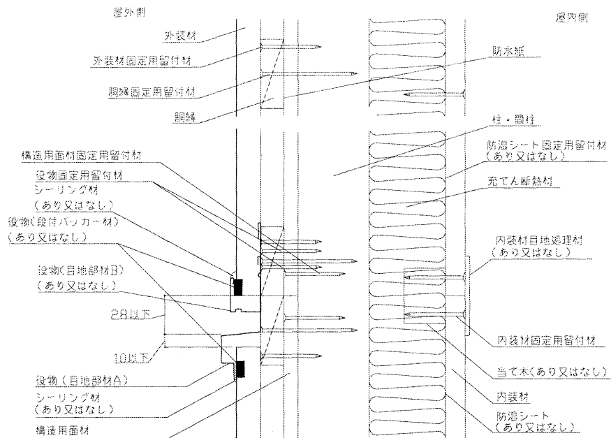
垂直断面図
