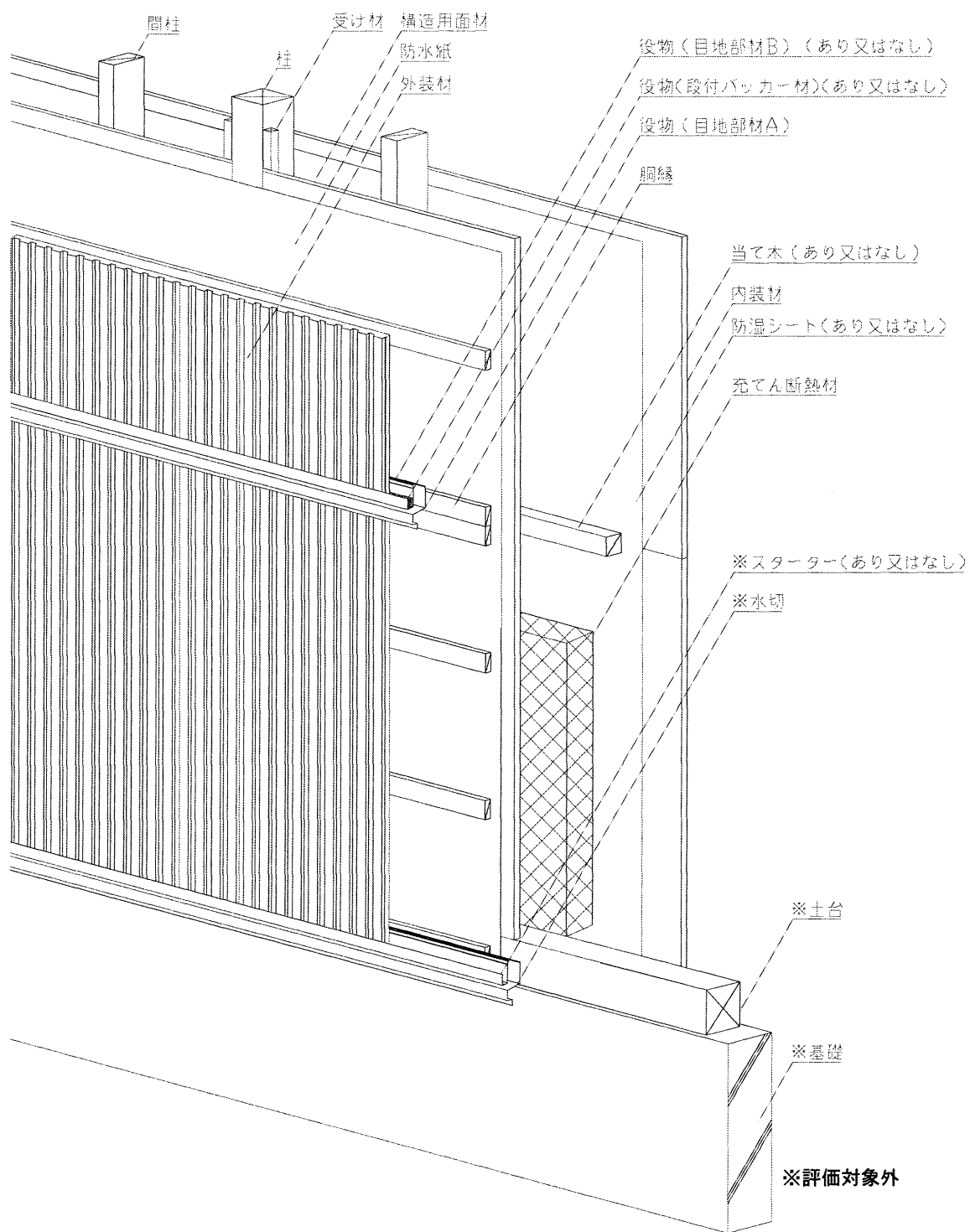
図1 構造説明図
