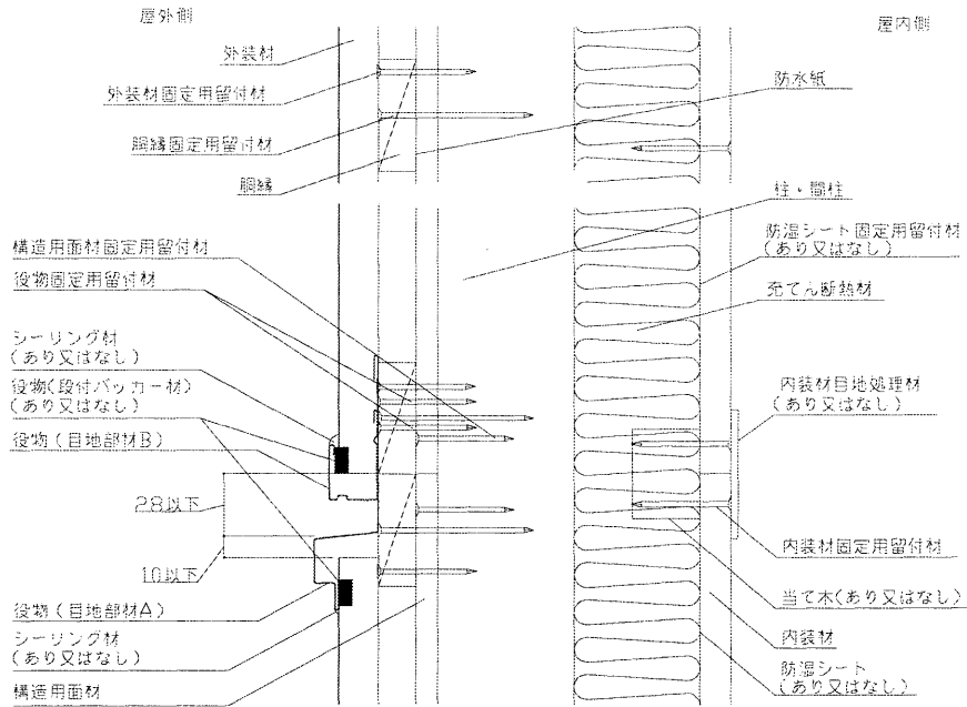
垂直断面図
