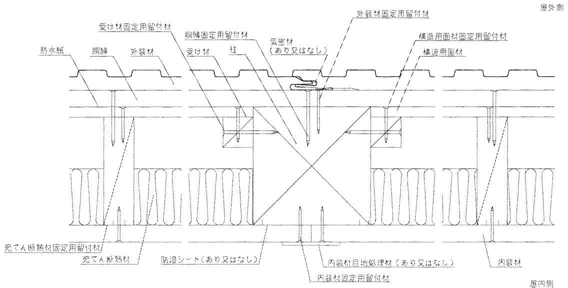
水平断面図
