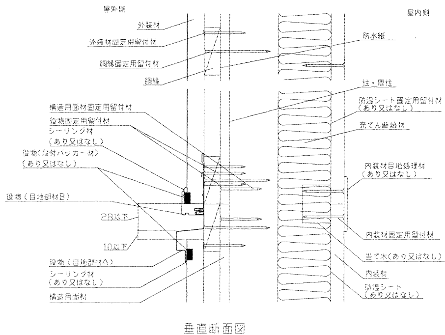
図5 構造説明図
