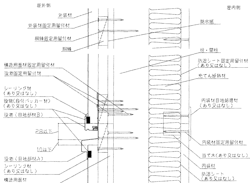
垂直断面図
