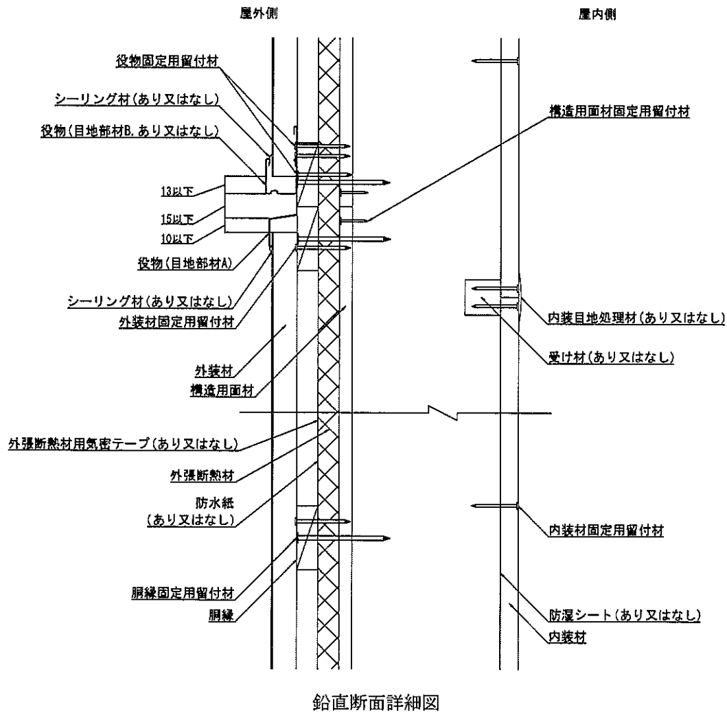
図2 構造説明図
