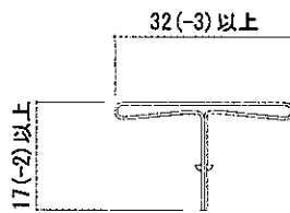
目地カバー(1ピースタイプ)
