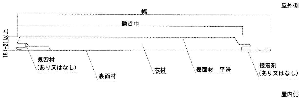
外装材断面
