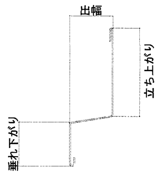
目地部材A 断面図(例)
