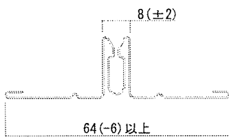
目地受け(鋼板製)
