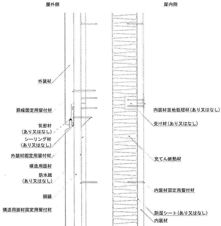
鉛直断面図
