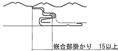
嵌合部詳細(例)
