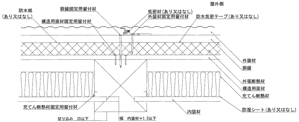
<水平断面図 面材：大壁、内装材：真壁-切り込み>
