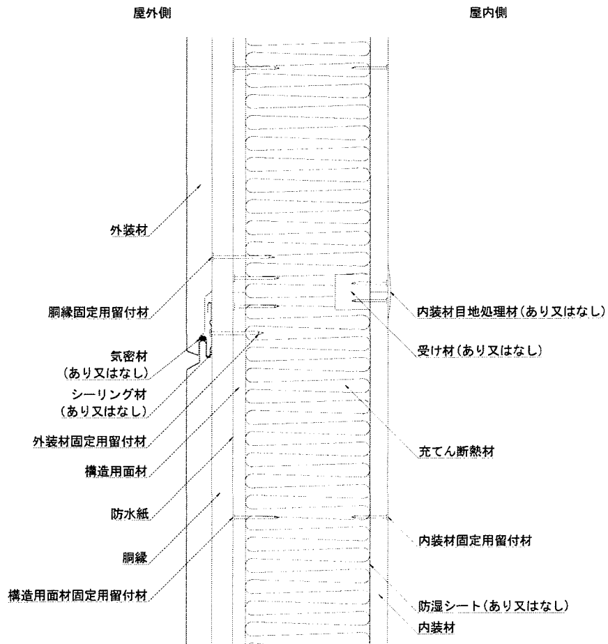
鉛直断面図
