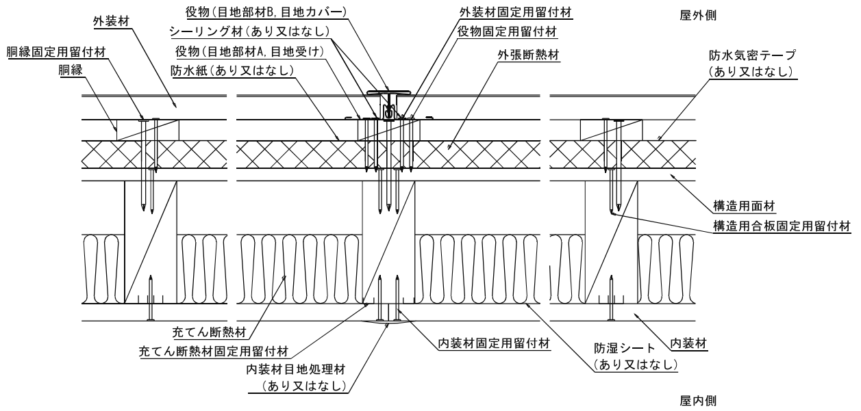
水平断面図
