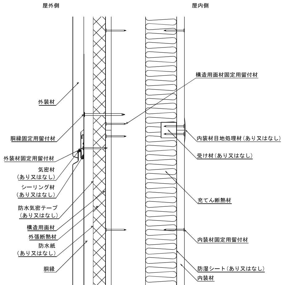
鉛直断面図
