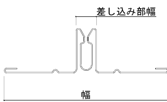
目地部材A(目地受け, 鋼板製)
