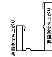
目地部材B(1ピースタイプ)
