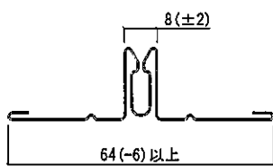
目地部材A(目地受け)
