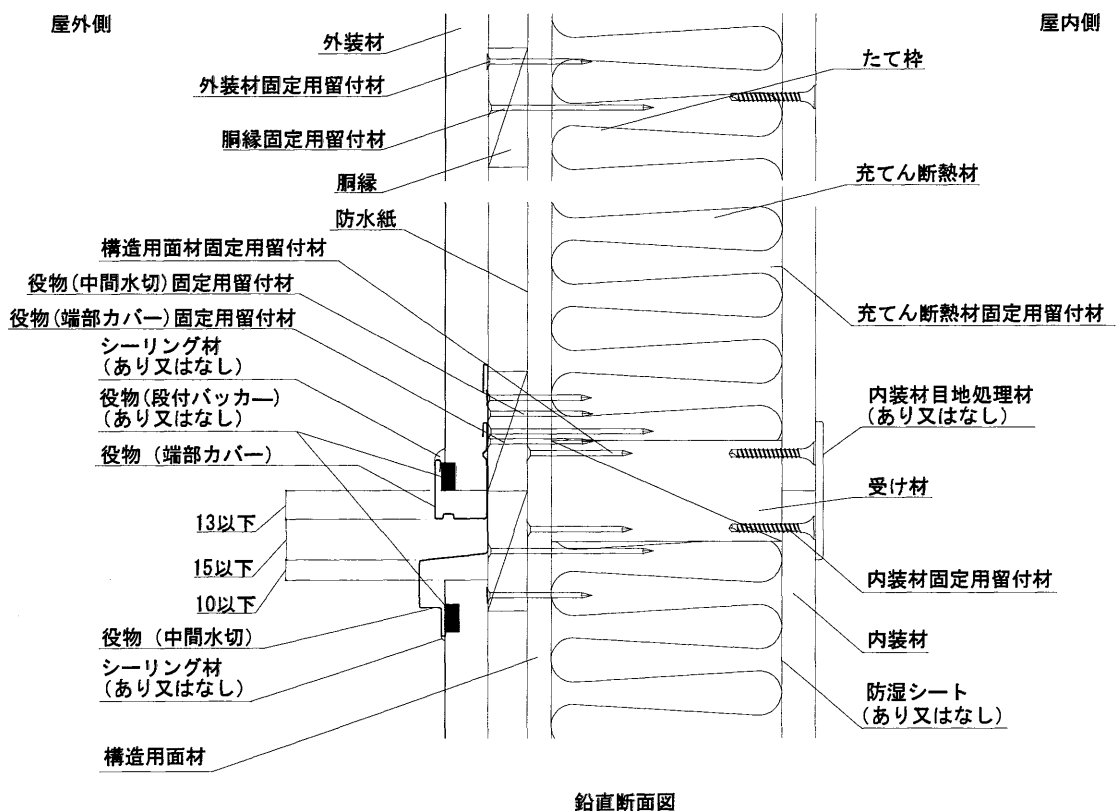
図2 構造説明図
