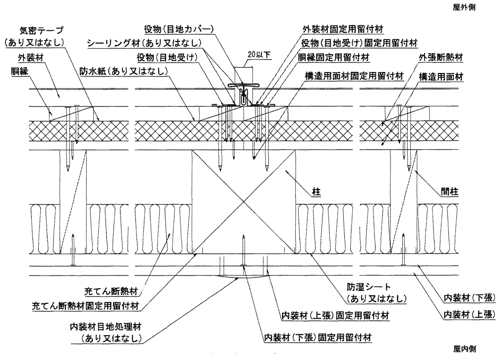
水平断面詳細図
