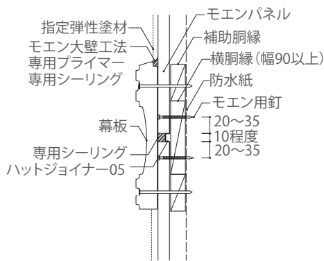
(横胴縁仕様の例)
