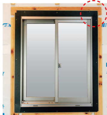
鋼板止水部材の上側T字部をサッシの上面に合わせる
