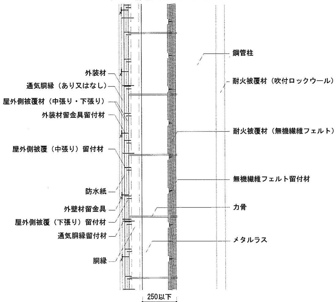
図3 構造説明図 (鉛直断面図)
