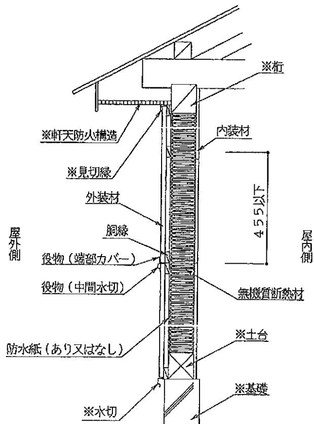
鉛直断面図
