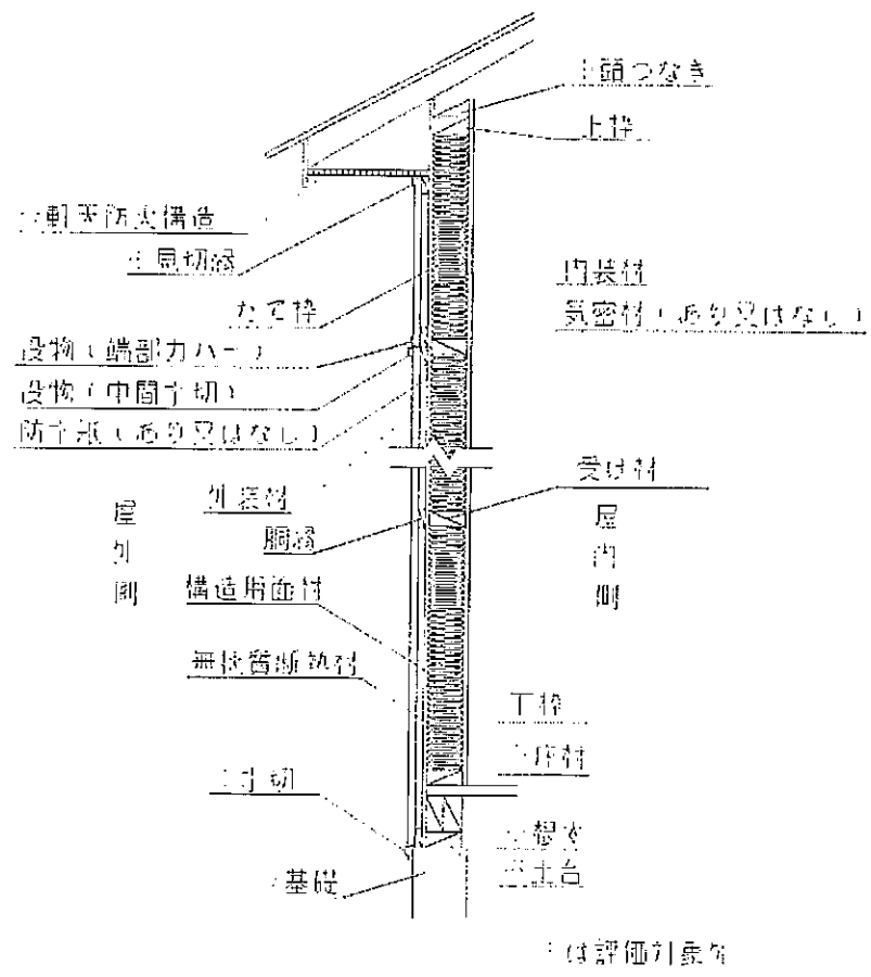
水平断面図
