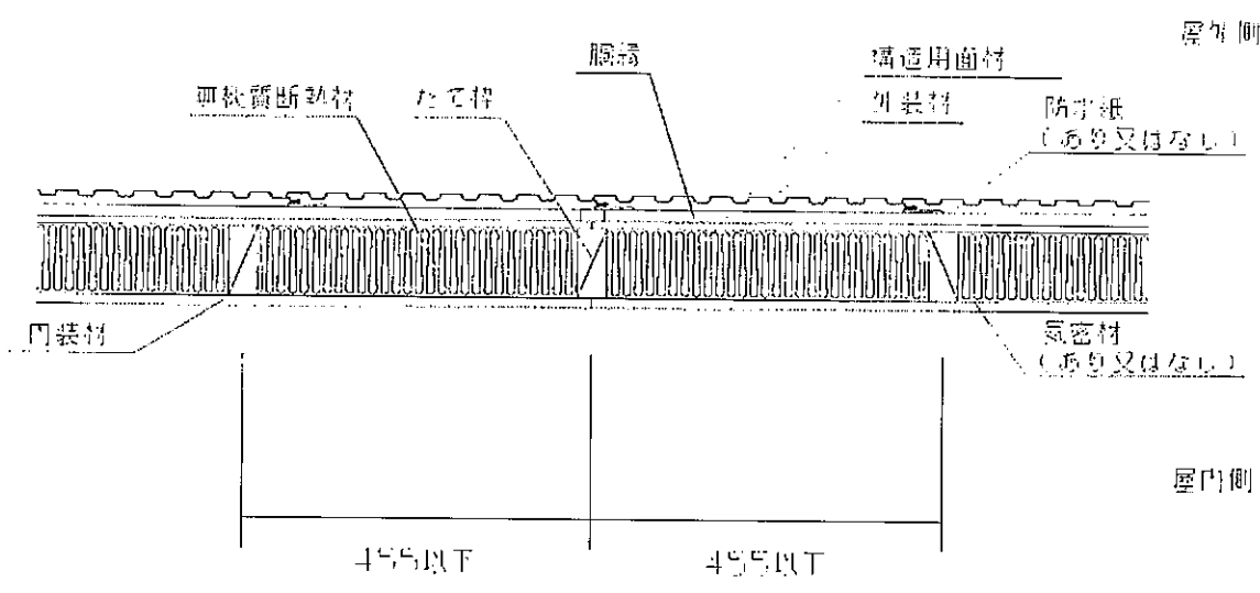
水平断面図
