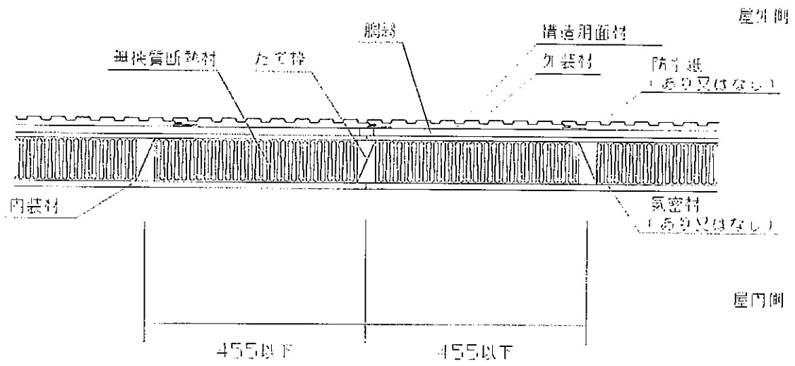
水平断面図
