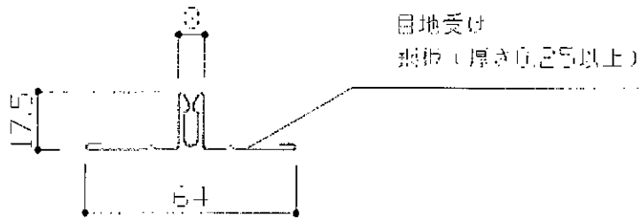
目地受け断面図
