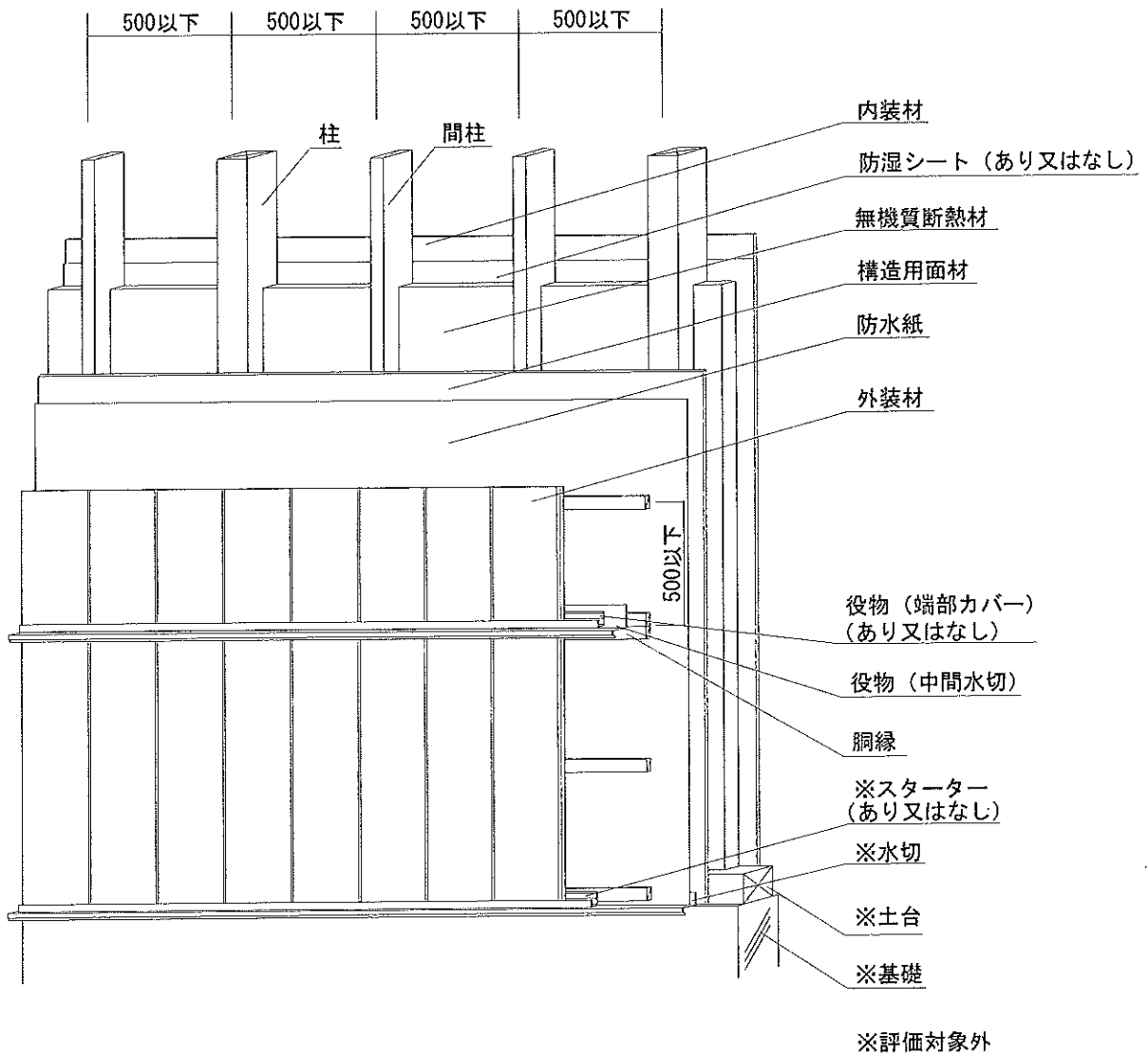
透視図
