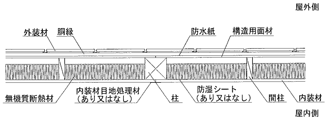
水平断面図
