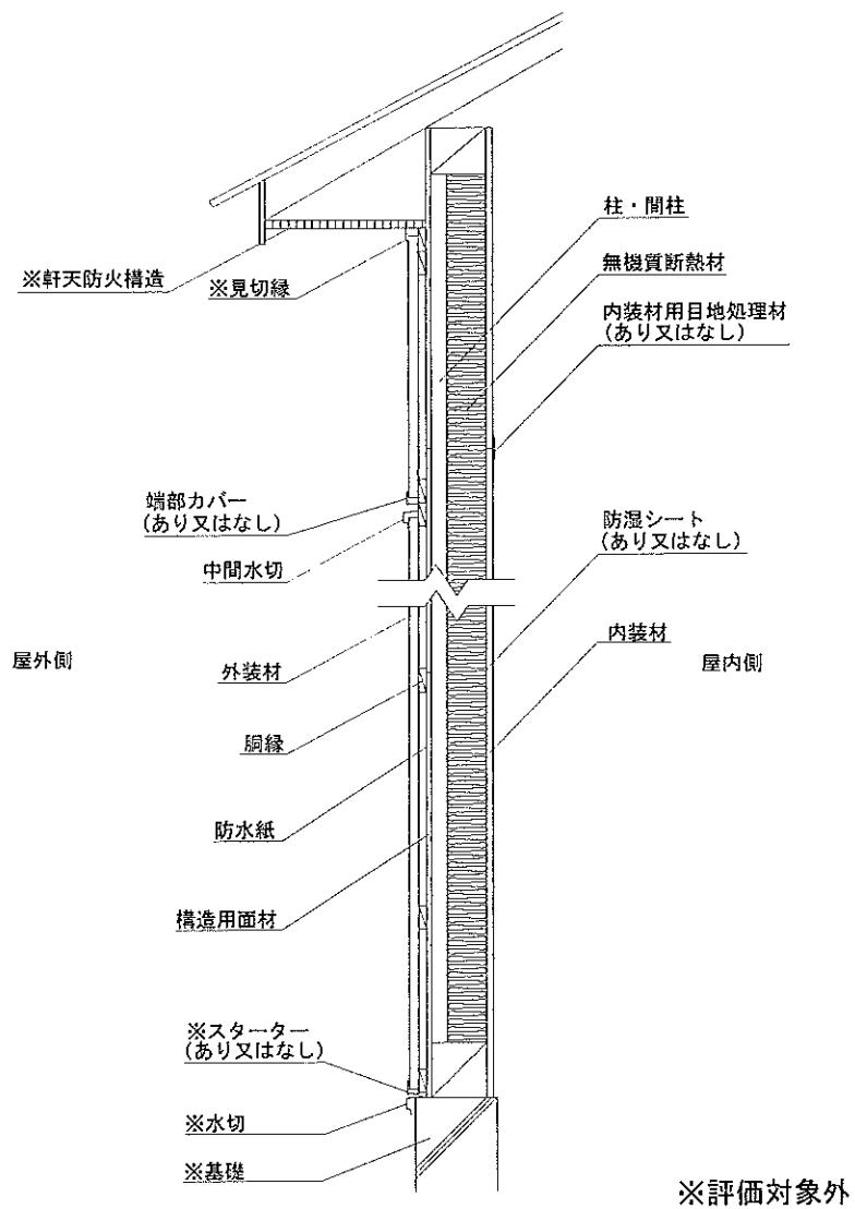
鉛直断面図
