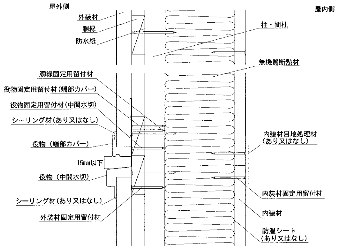
鉛直断面図
