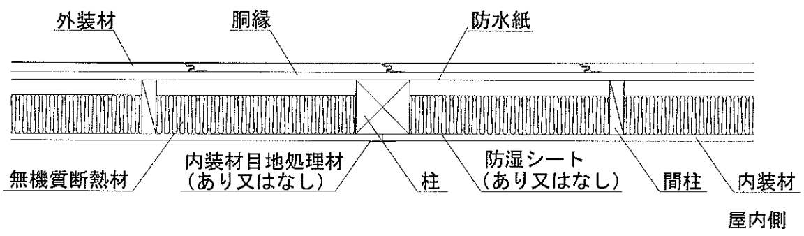
水平断面図
