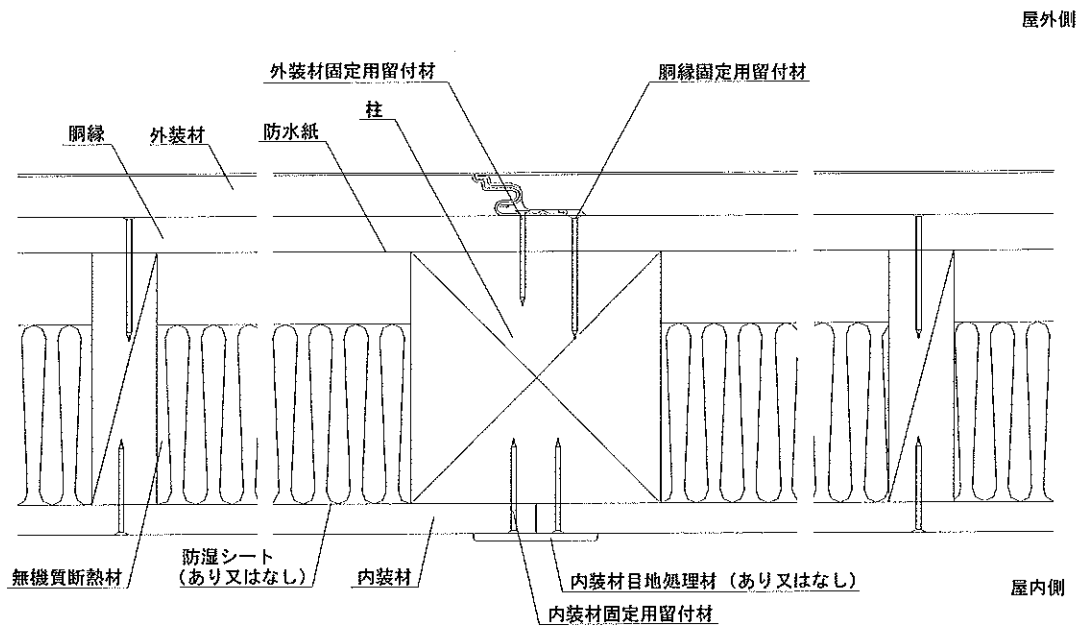
水平断面図
