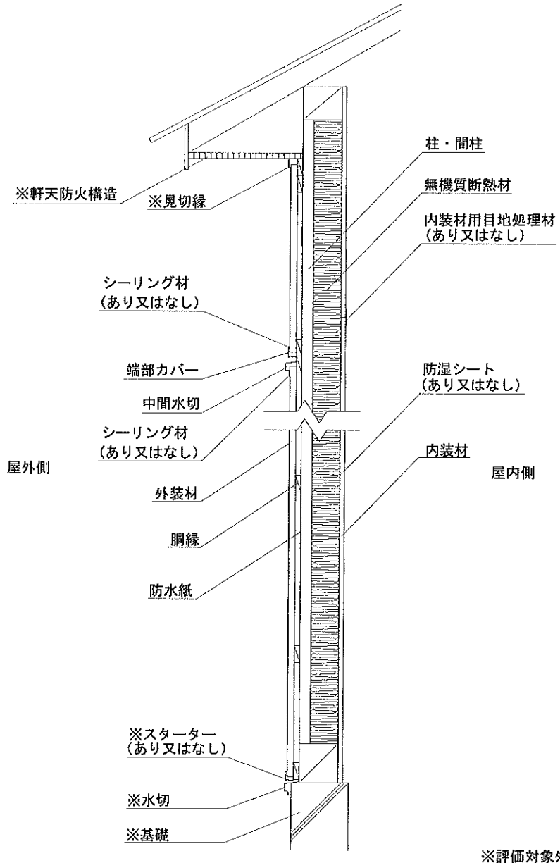
鉛直断面図
