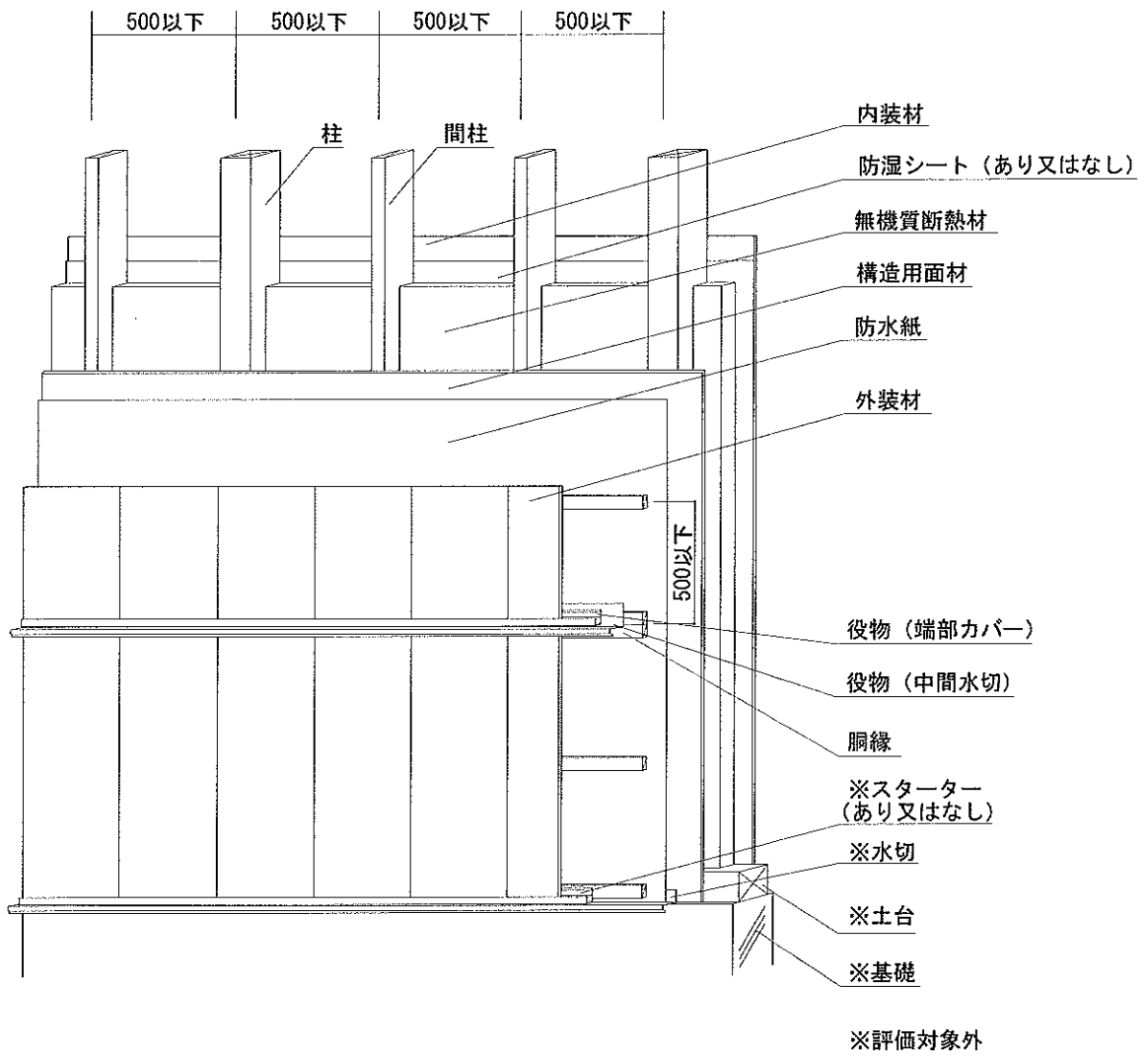
透視図
