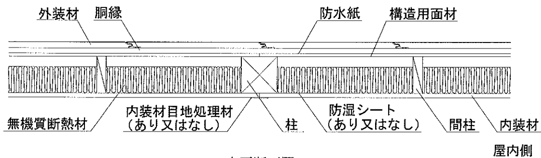
水平断面図
