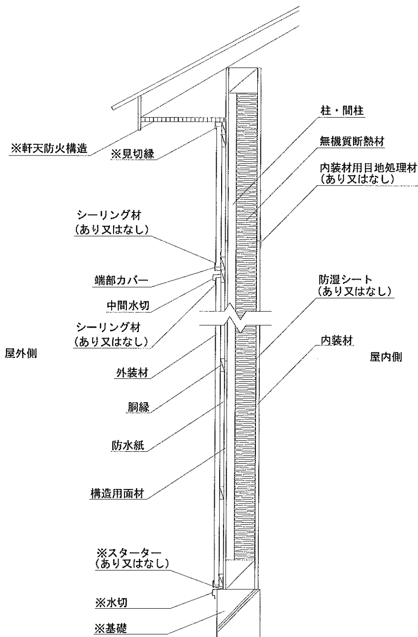
鉛直断面図
