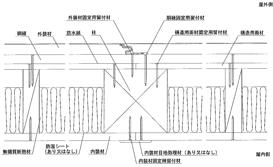
水平断面図
