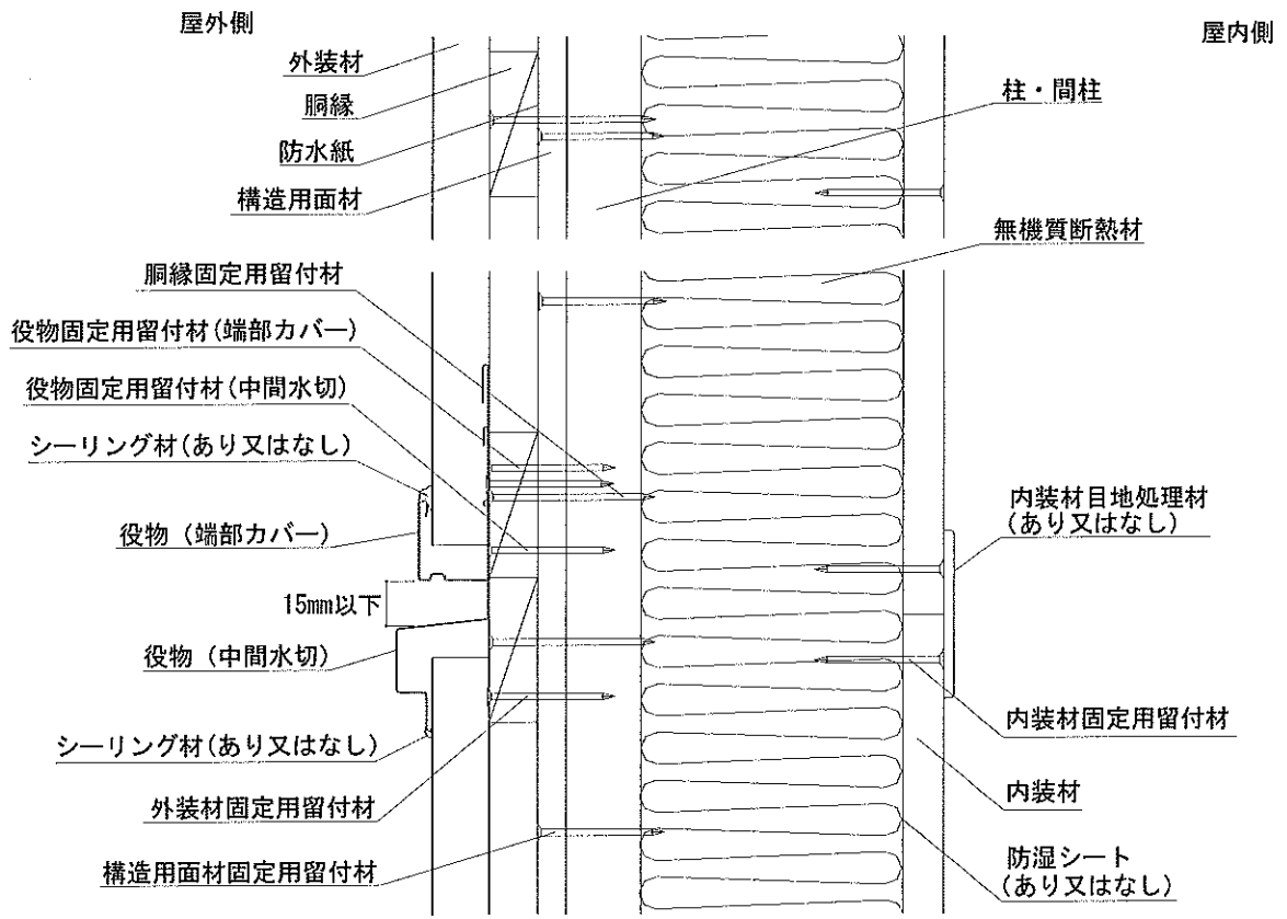
鉛直断面図
