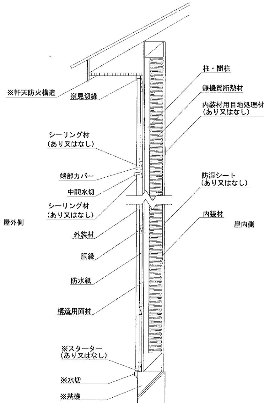
鉛直断面図
