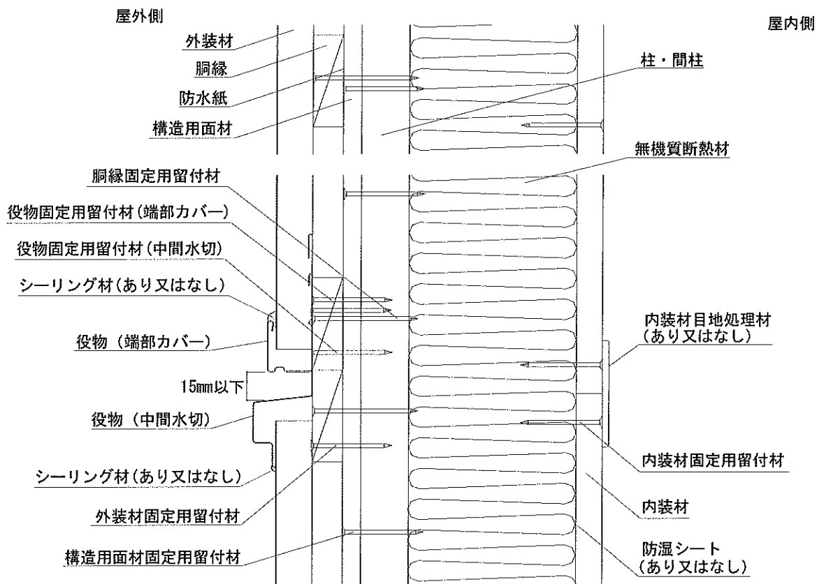
鉛直断面図
