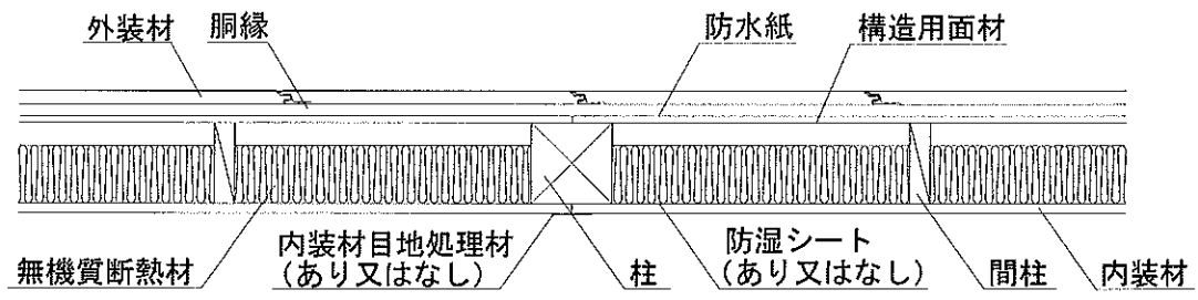
水平断面図
