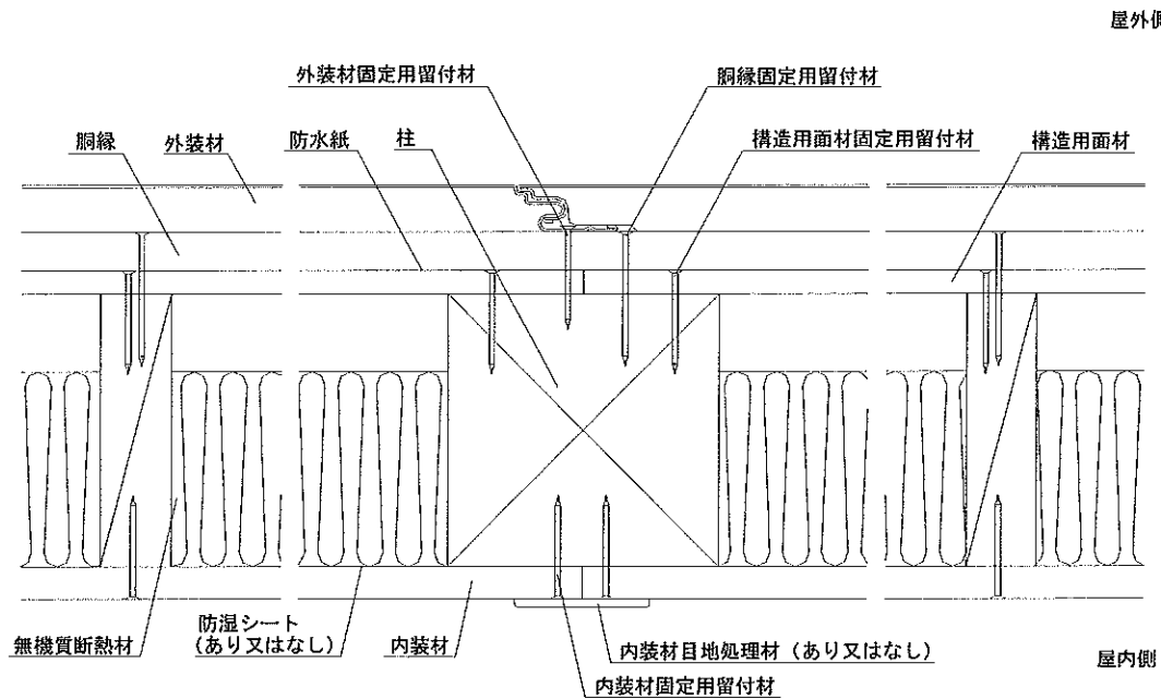
水平断面図
