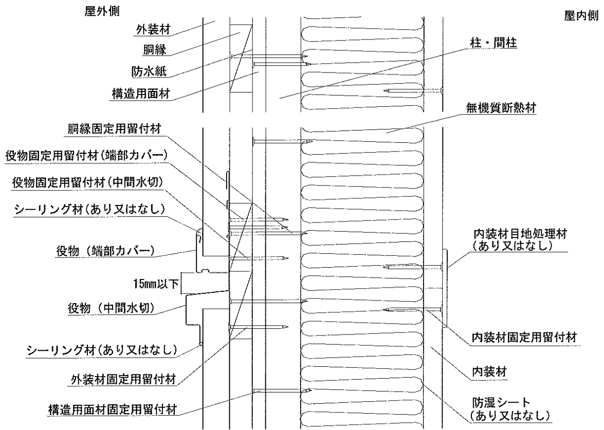
鉛直断面図
