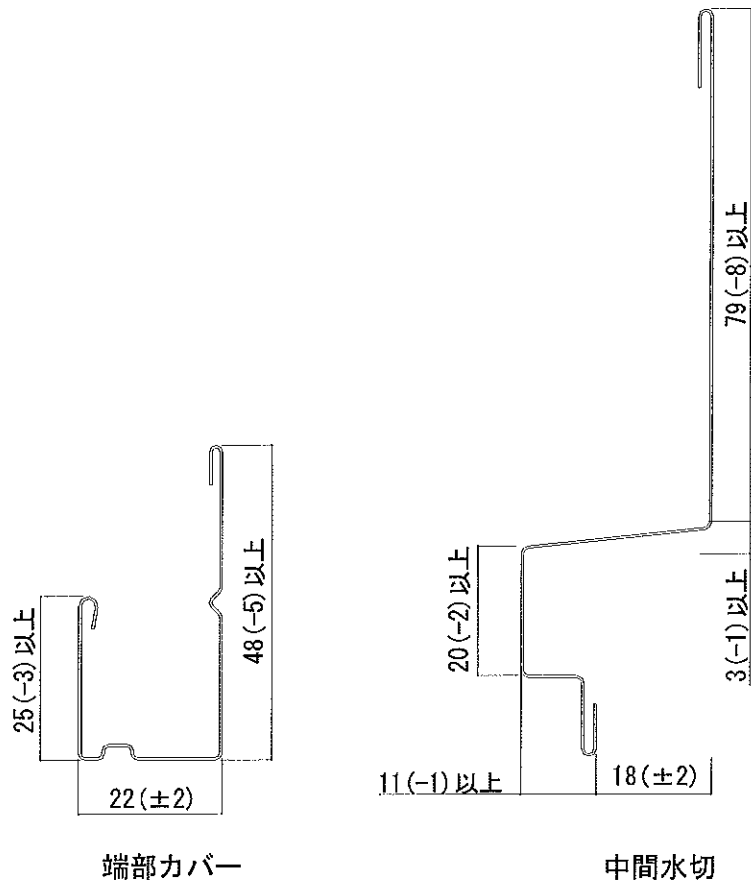
図4 役物形状図
