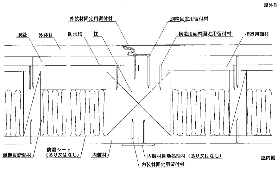
水平断面図
