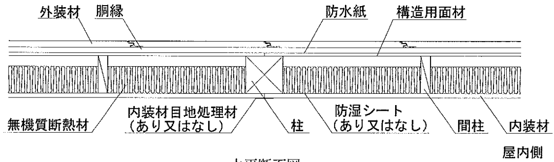
水平断面図
