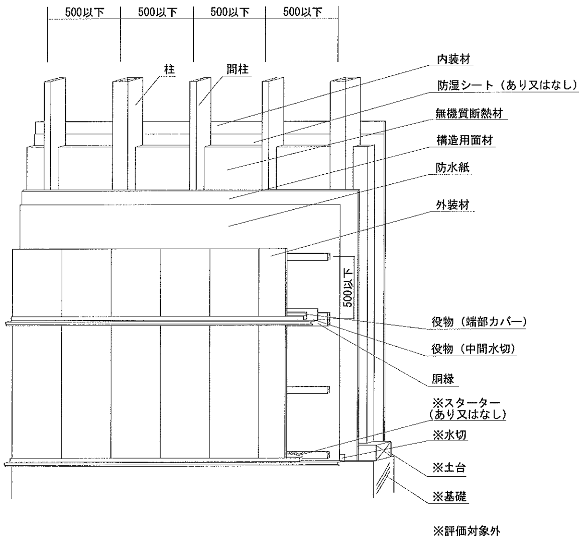
透視図
