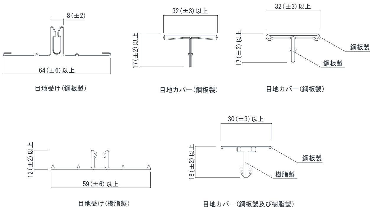
役物断面図
