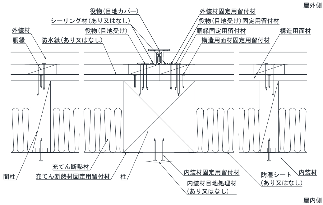
水平断面図
