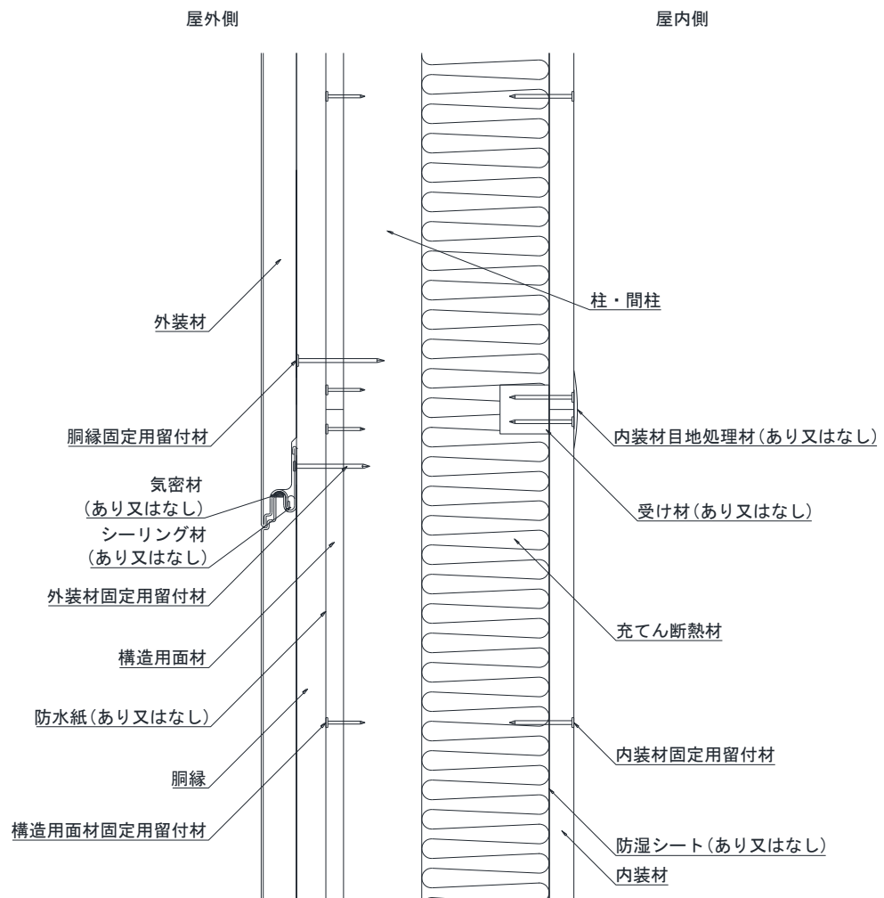
鉛直断面図
