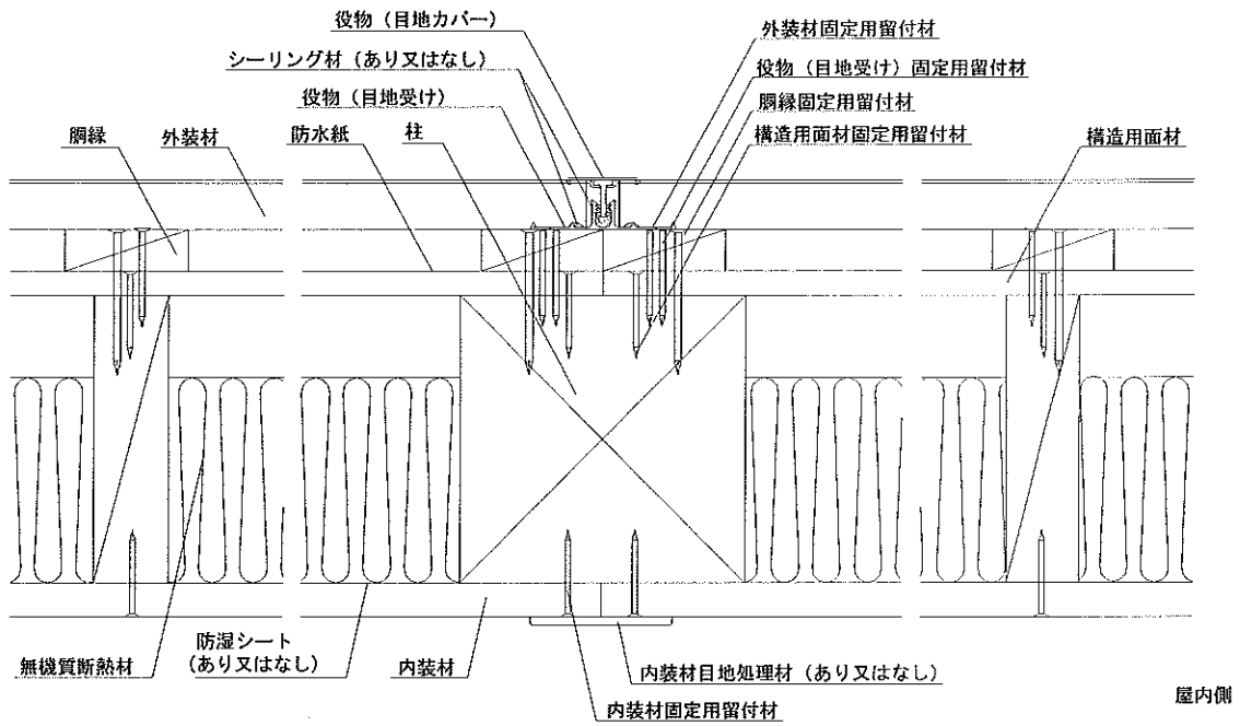
水平断面図
