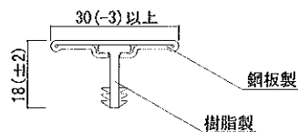
目地カバー (鋼板及び樹脂製)
