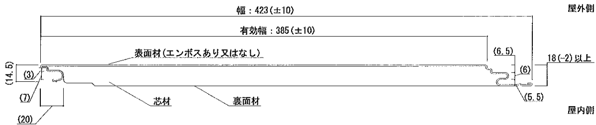
外装材形状図
