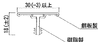
目地カバー(鋼板及び樹脂製)
