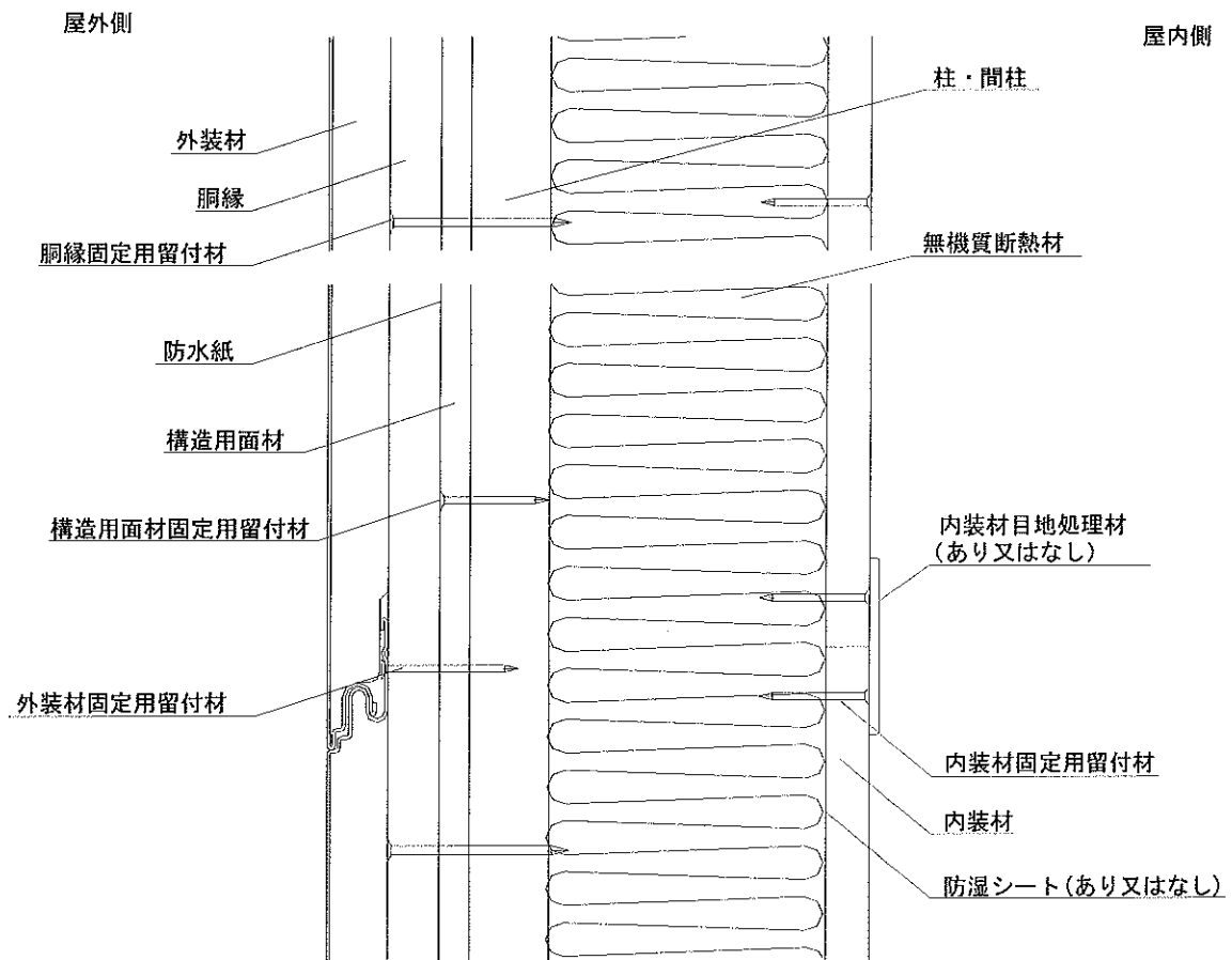
鉛直断面図 図2 構造説明図
