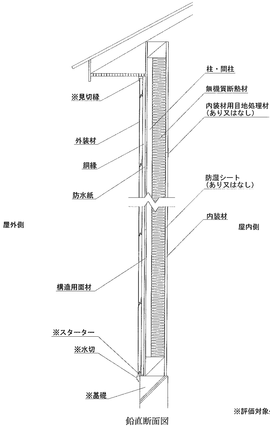
図4 施工図
