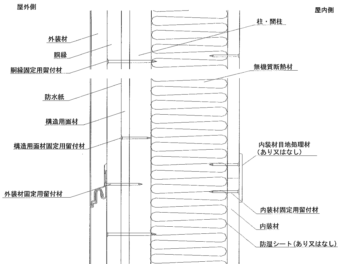
鉛直断面図
