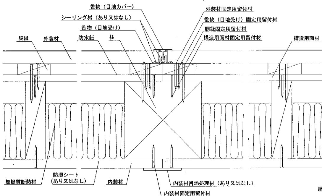
水平断面図
