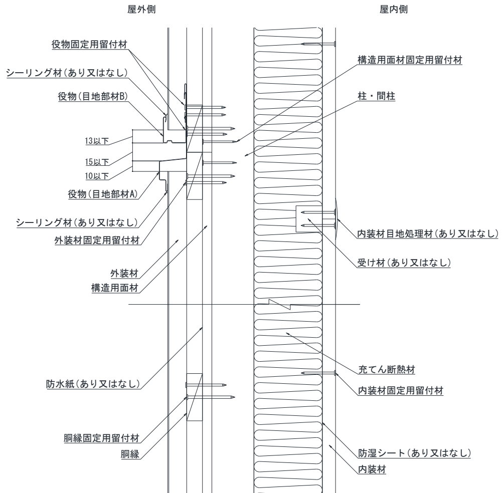
鉛直断面図
