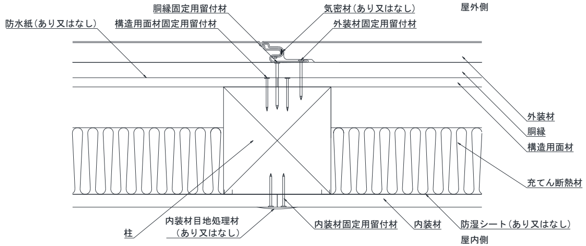
水平断面図
