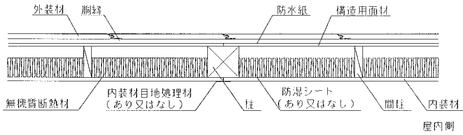
水平断面図
