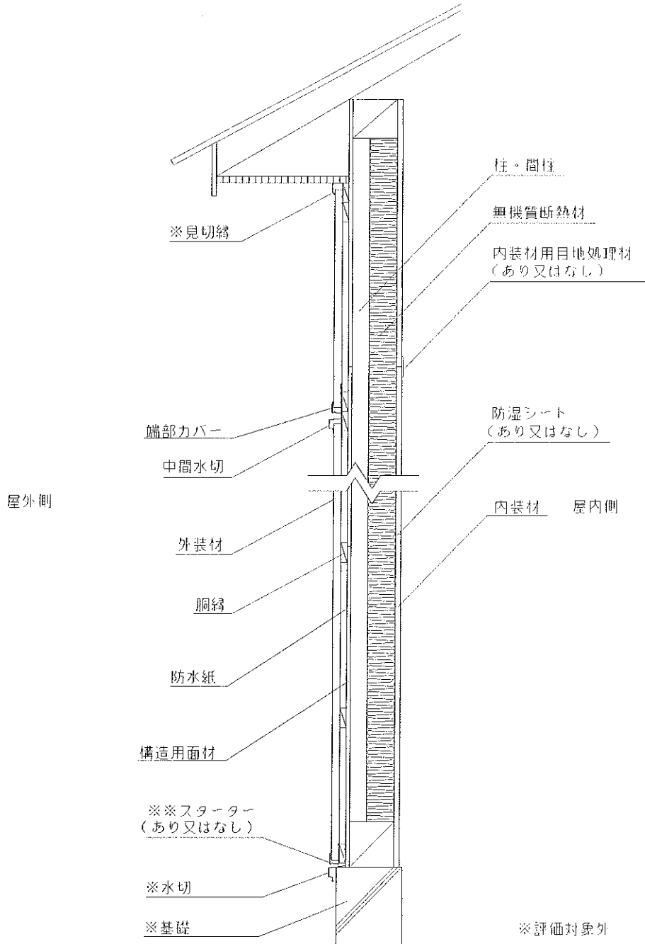
鉛直断面図
