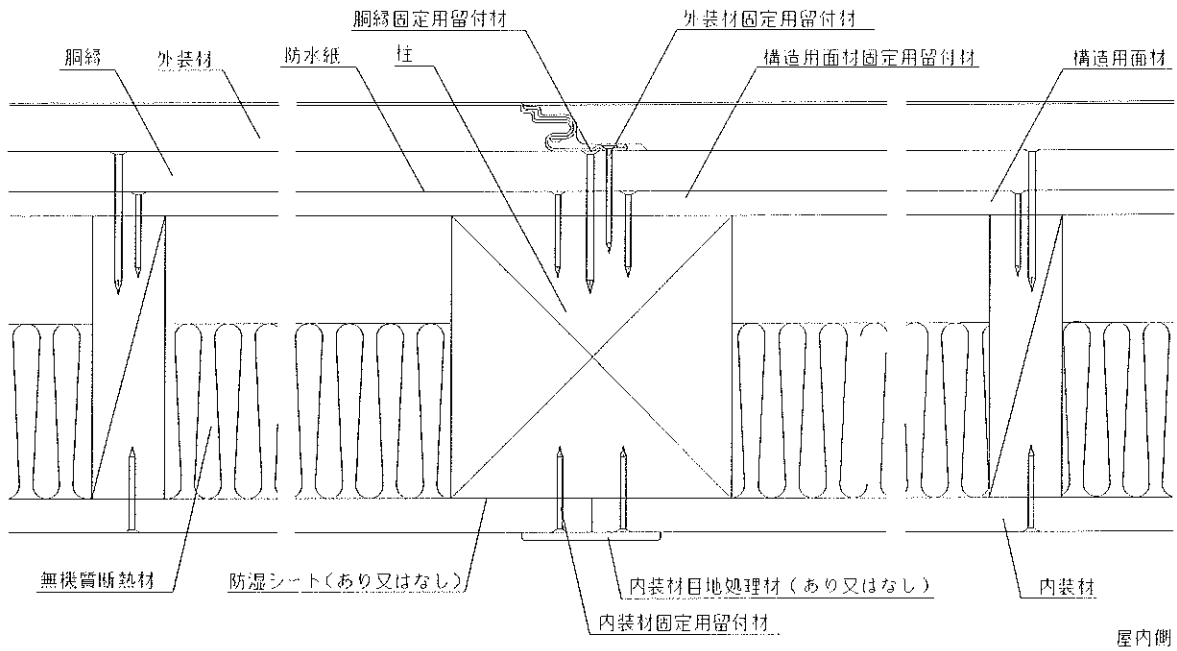
水平断面図
