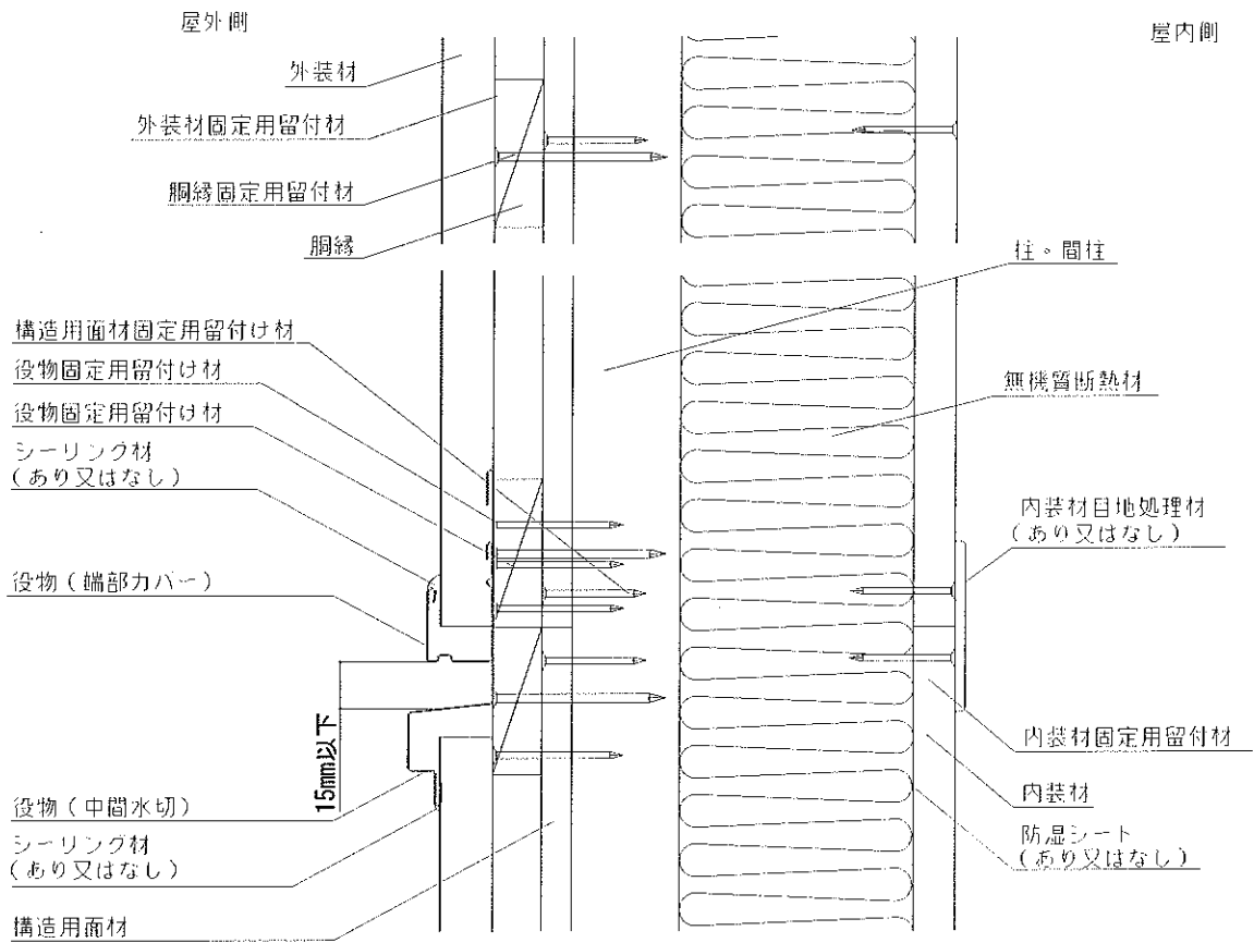
鉛直断面図
