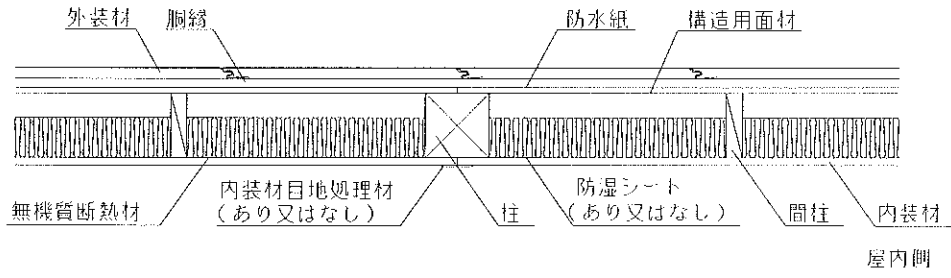
水平断面図
