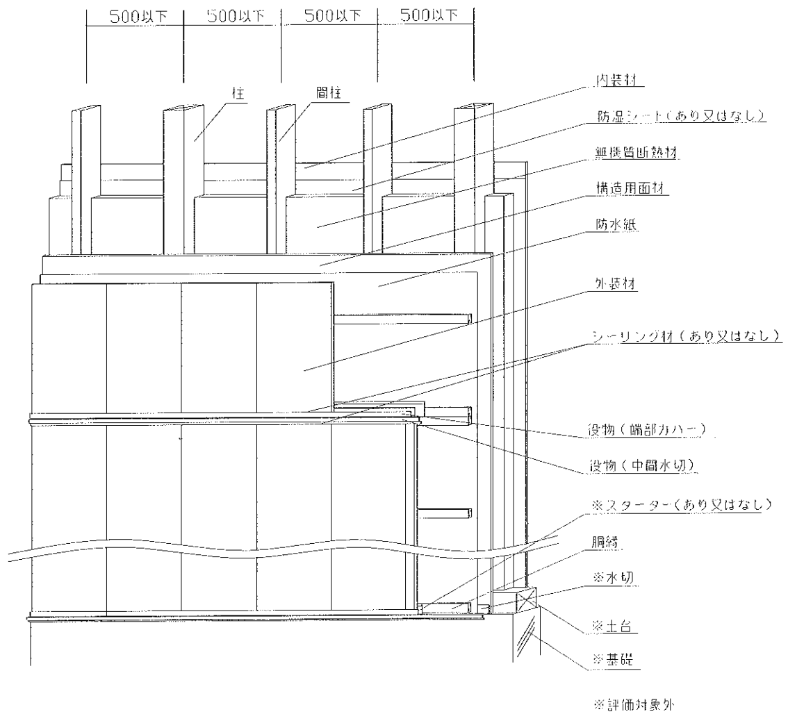
透視図
