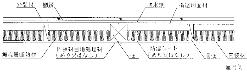
水平断面図
