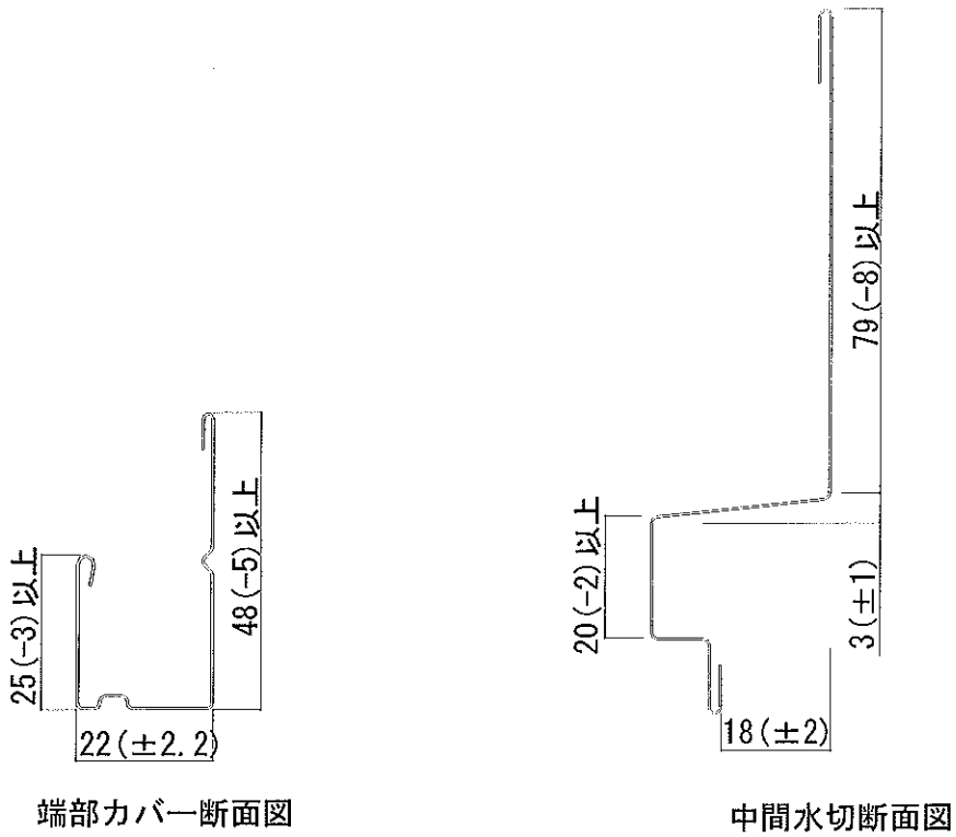
役物形状図
