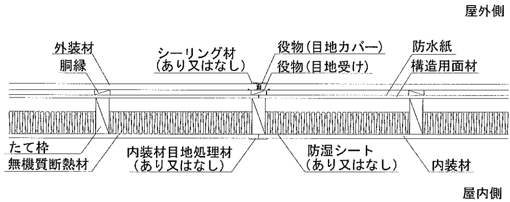
水平断面図
