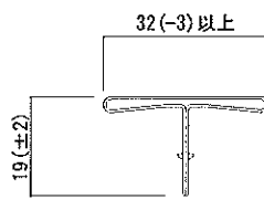
目地カバー(鋼板製)
