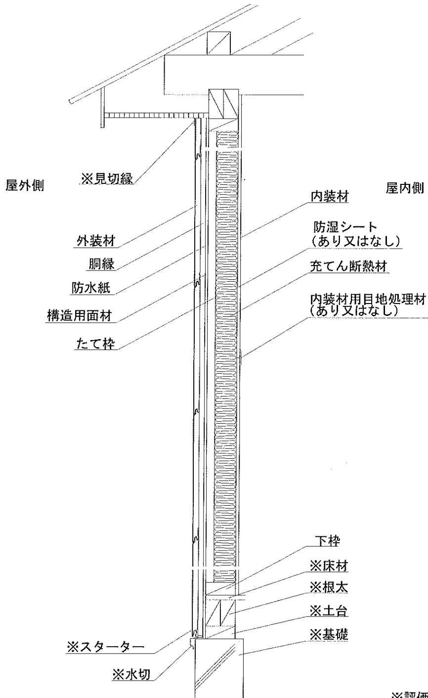
図4 施工図
