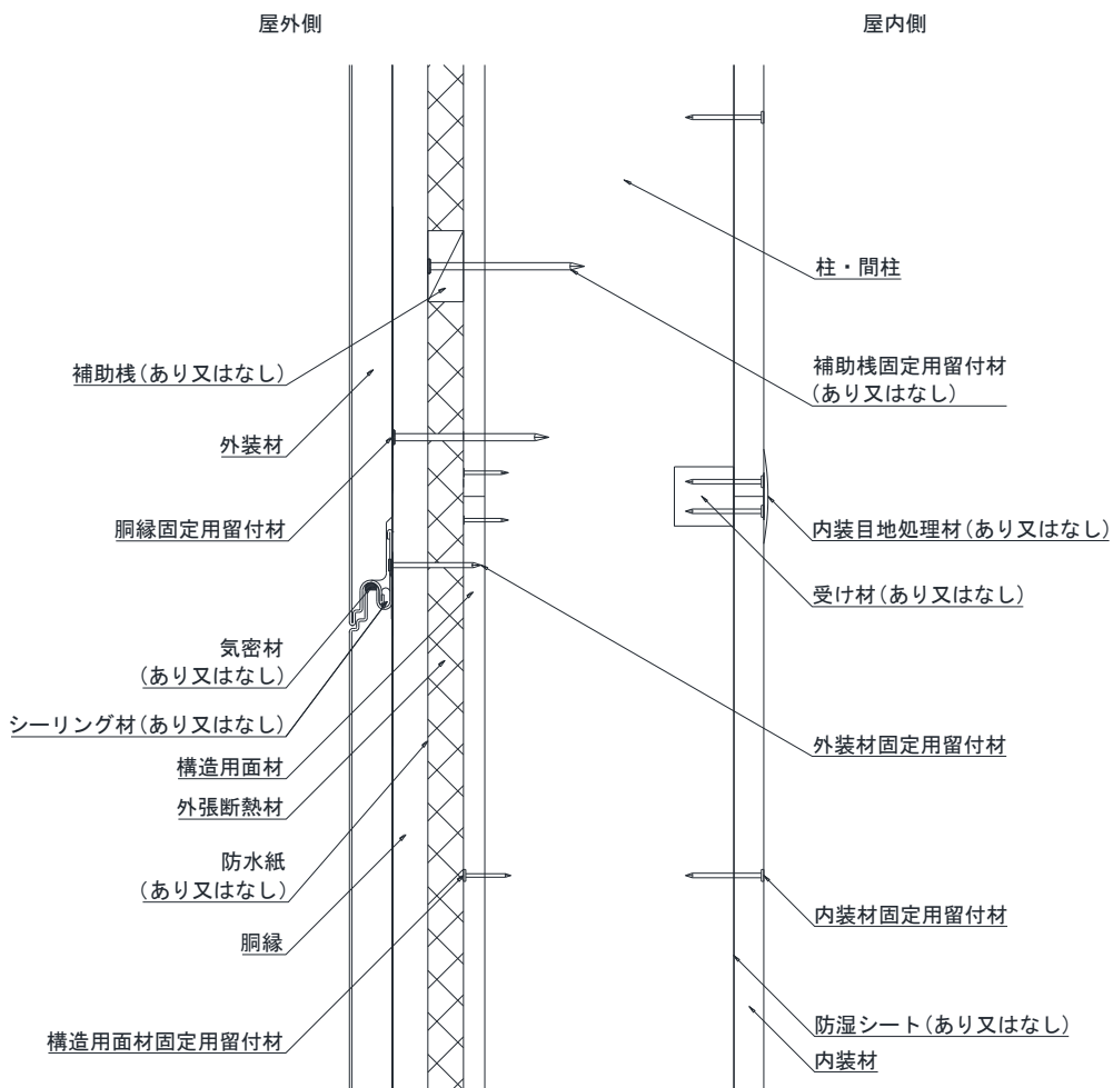
鉛直断面図 (充てん断熱材なし) 図2 構造説明図
