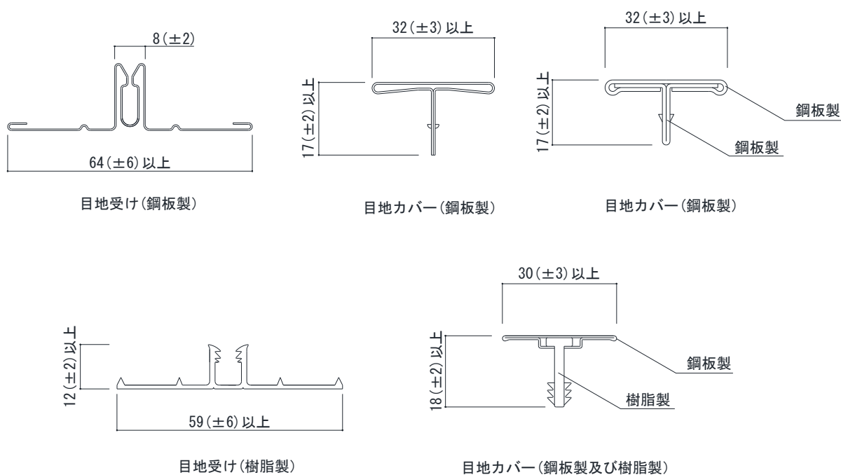
役物断面図
