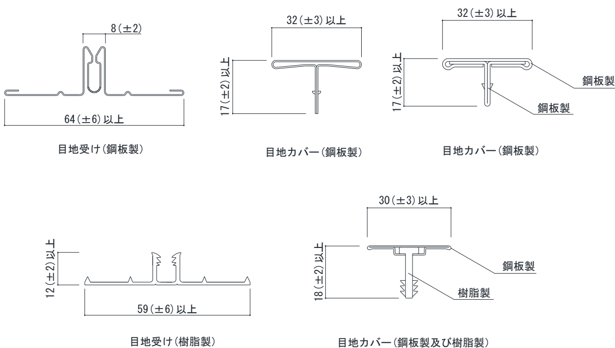
役物断面図
