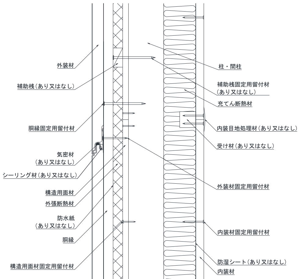
鉛直断面図 (充てん断熱材あり) 図2 構造説明図
