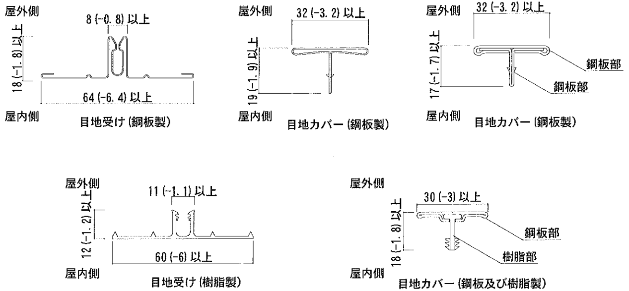
役物断面図
