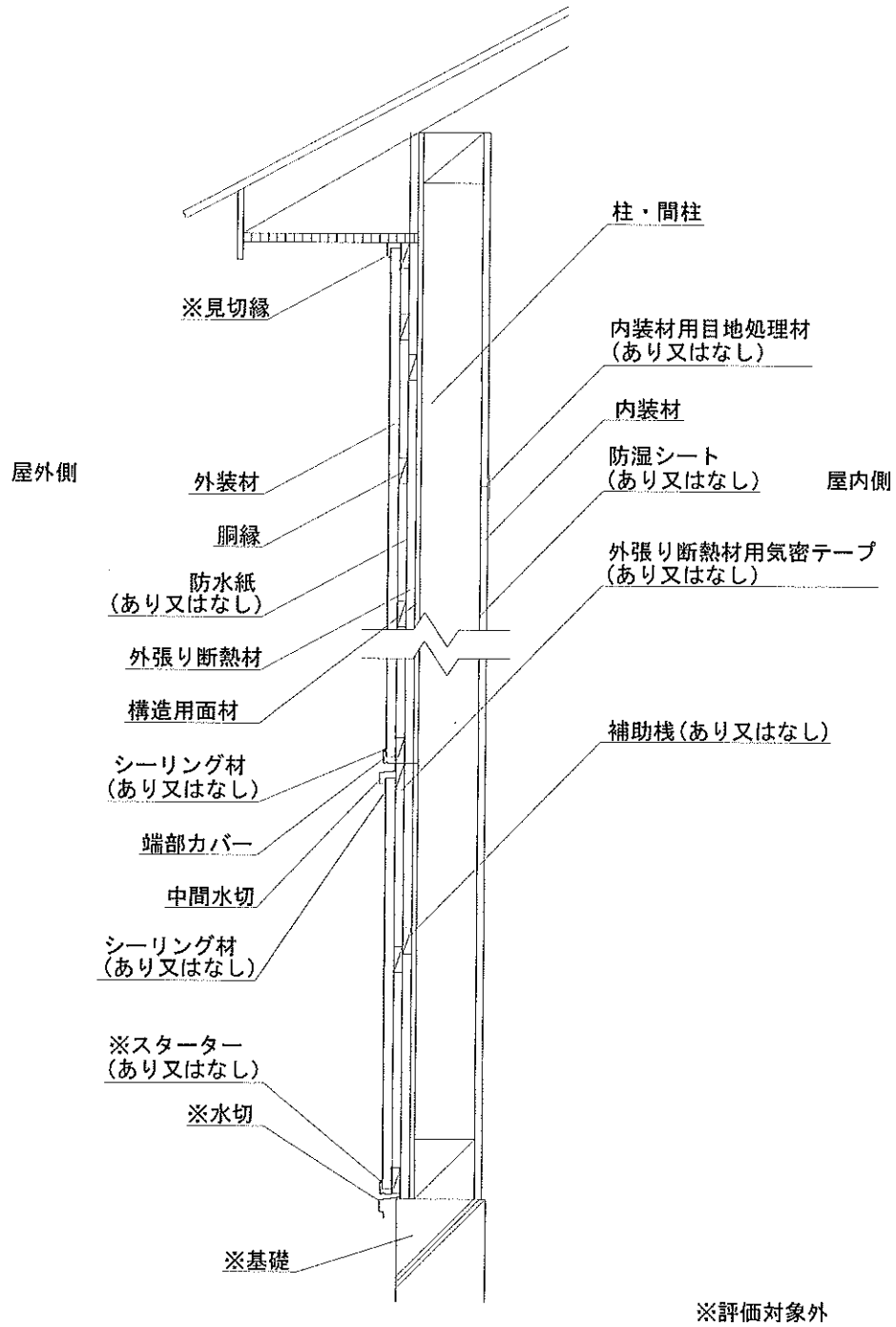
図4 施工図
