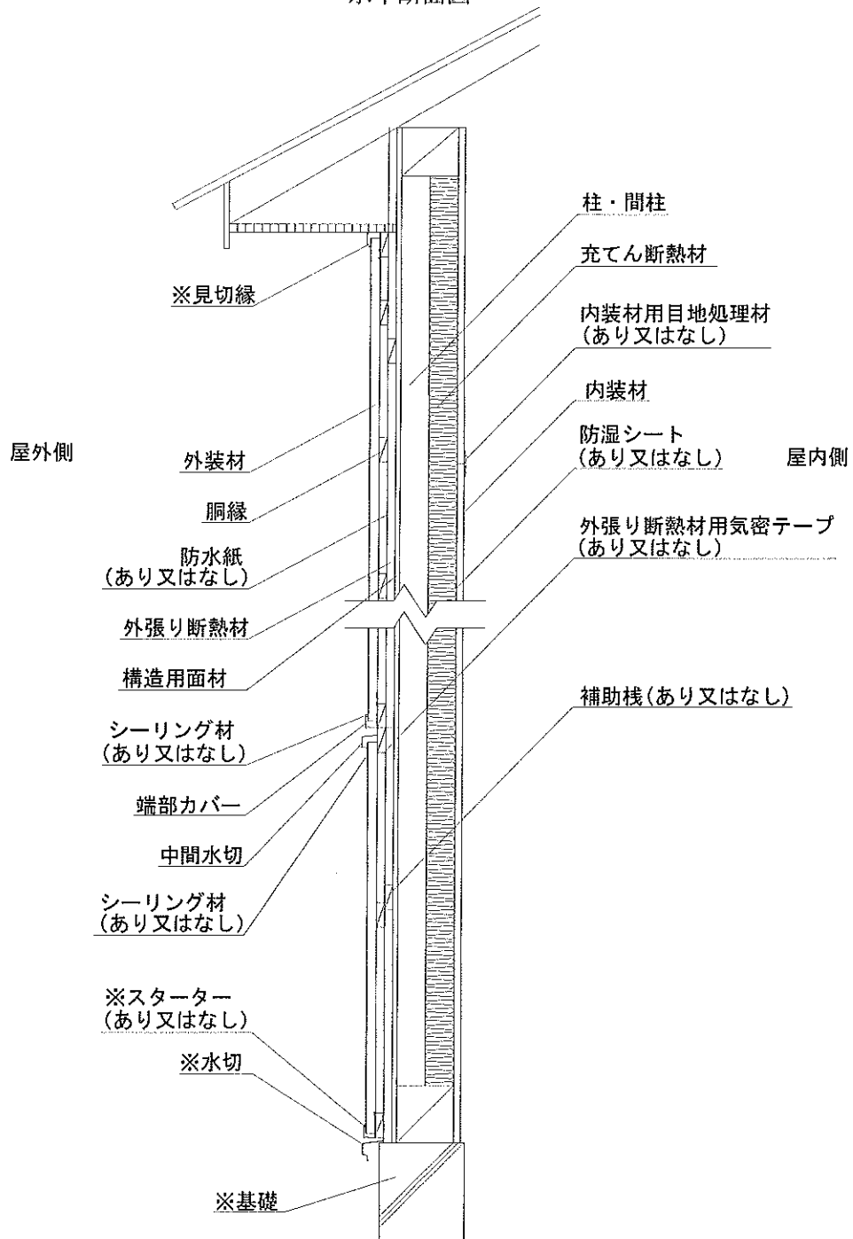
鉛直断面図
