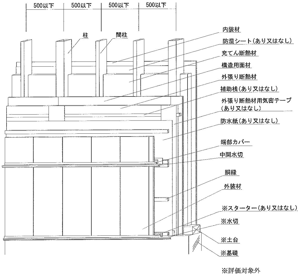
透視図
