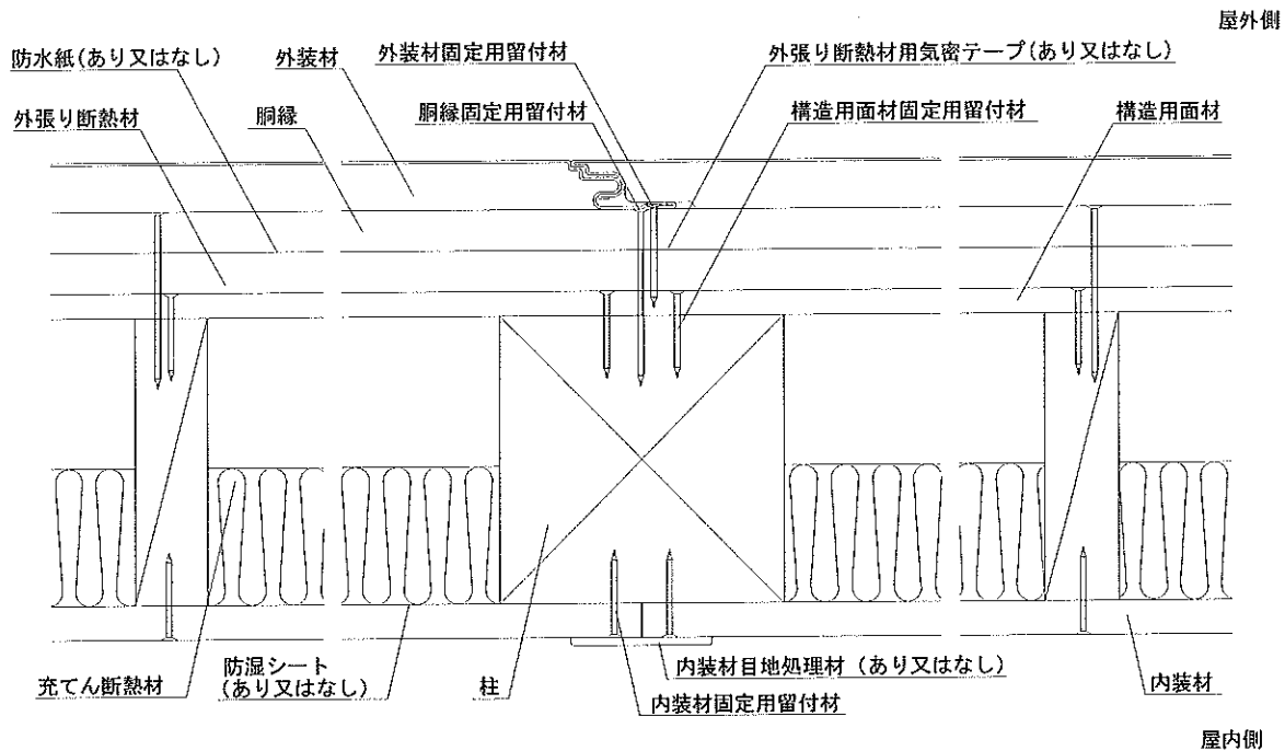
水平断面図
