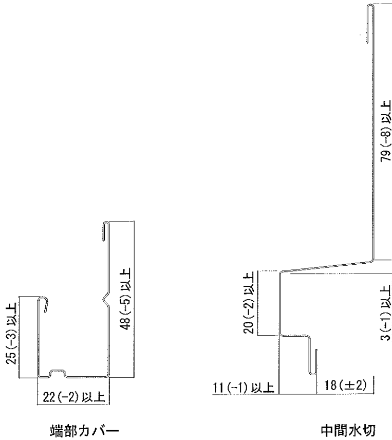
図3 構造説明図
