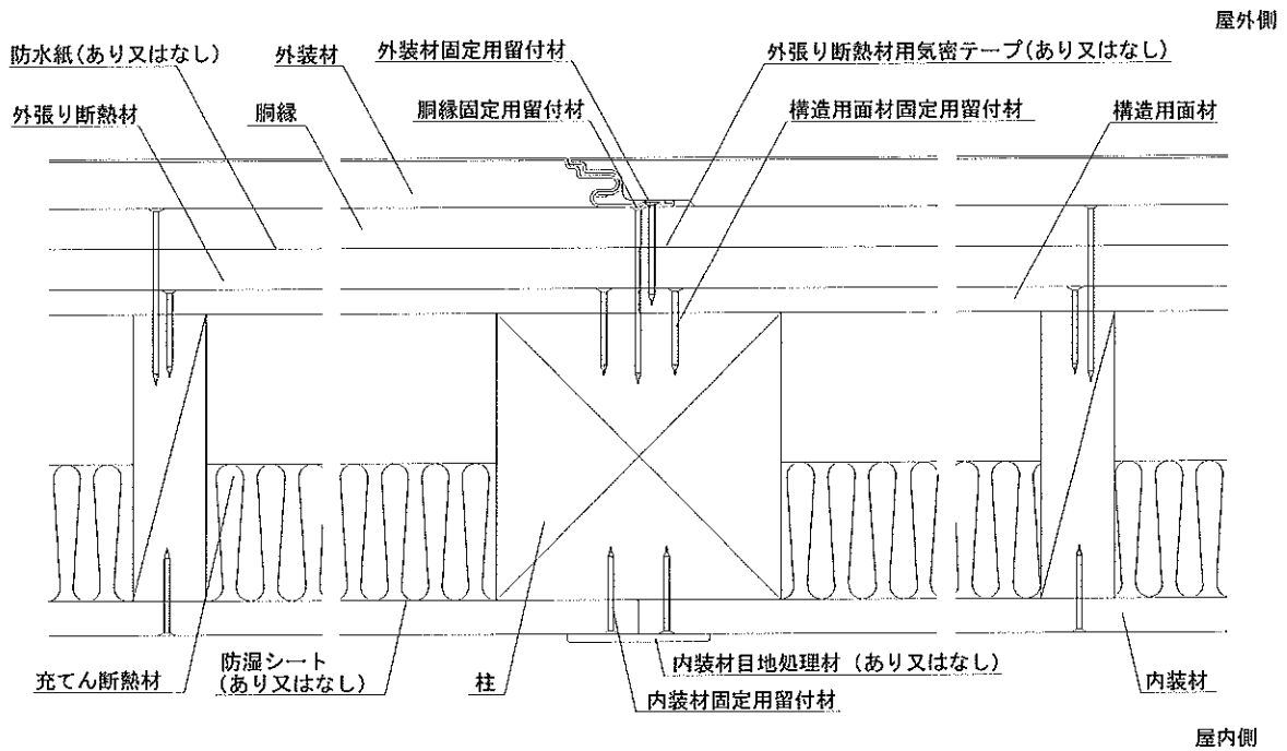
水平断面図
