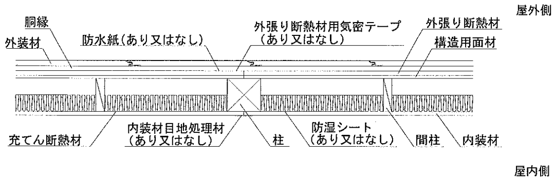
水平断面図
