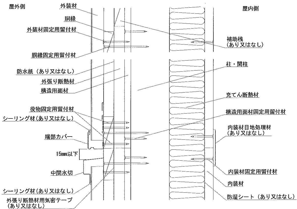
鉛直断面図
