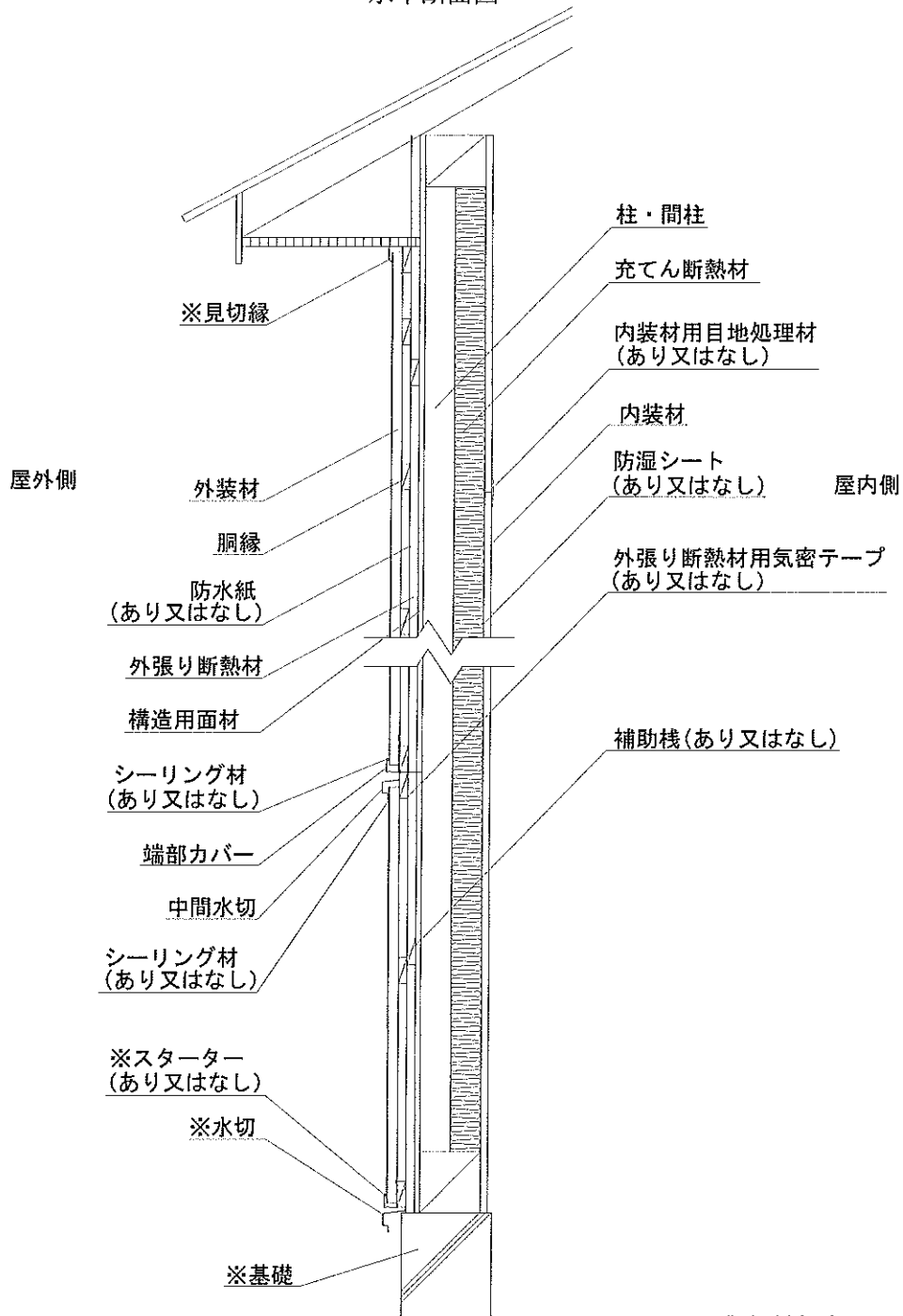
鉛直断面図
