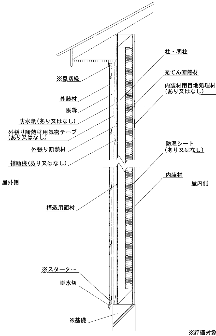
鉛直断面図
