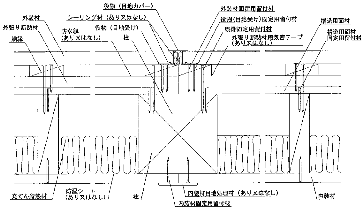
水平断面図
