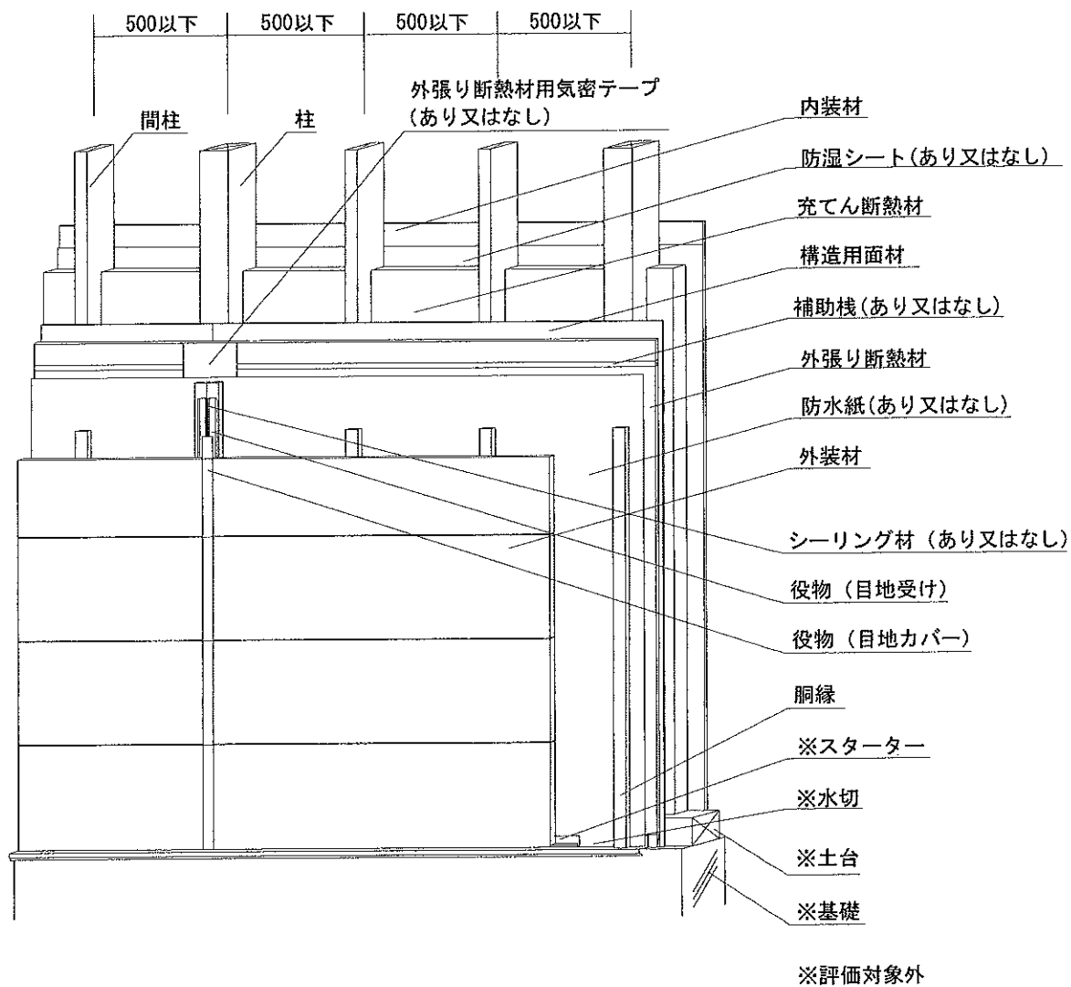
透視図
