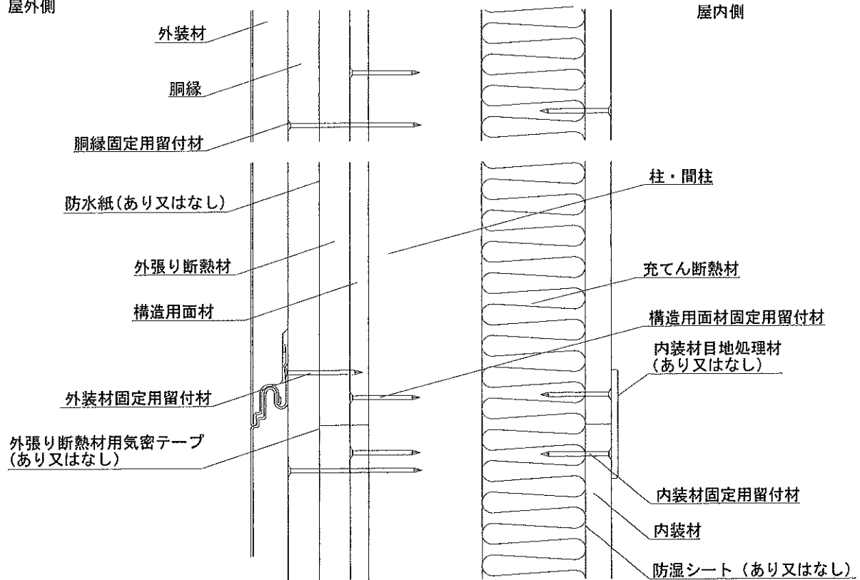
鉛直断面図
