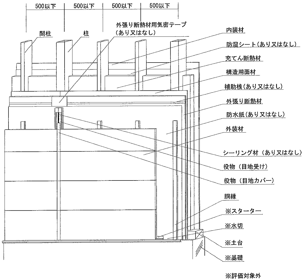
透視図
