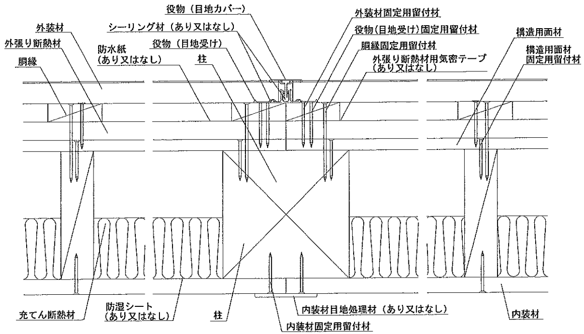
水平断面図
