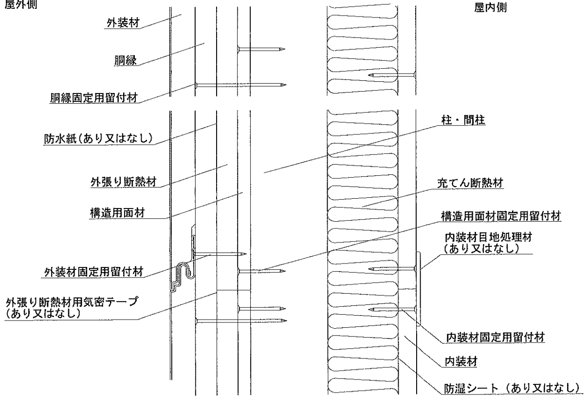
鉛直断面図
