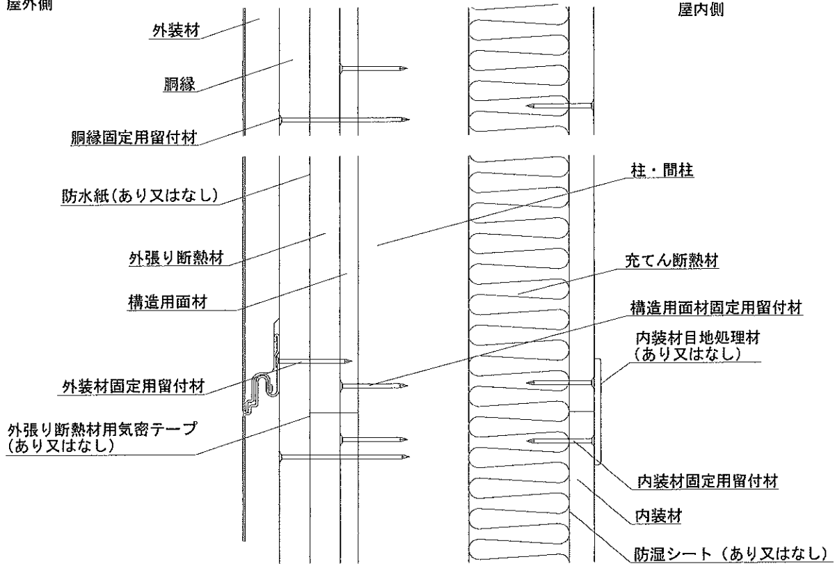
鉛直断面図
