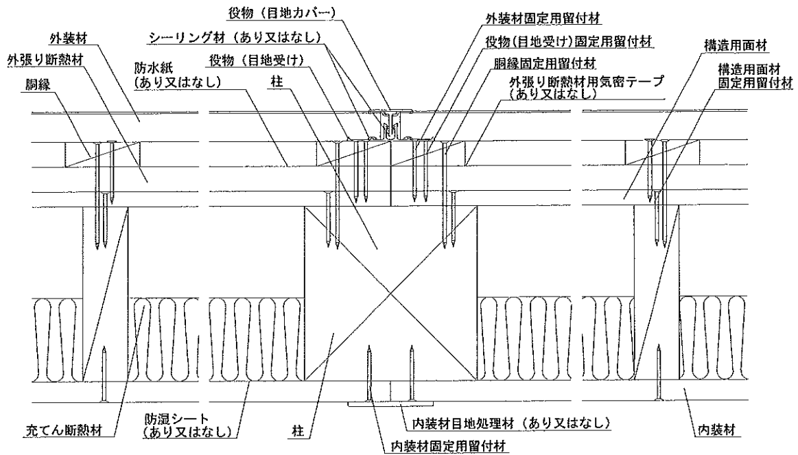
水平断面図
