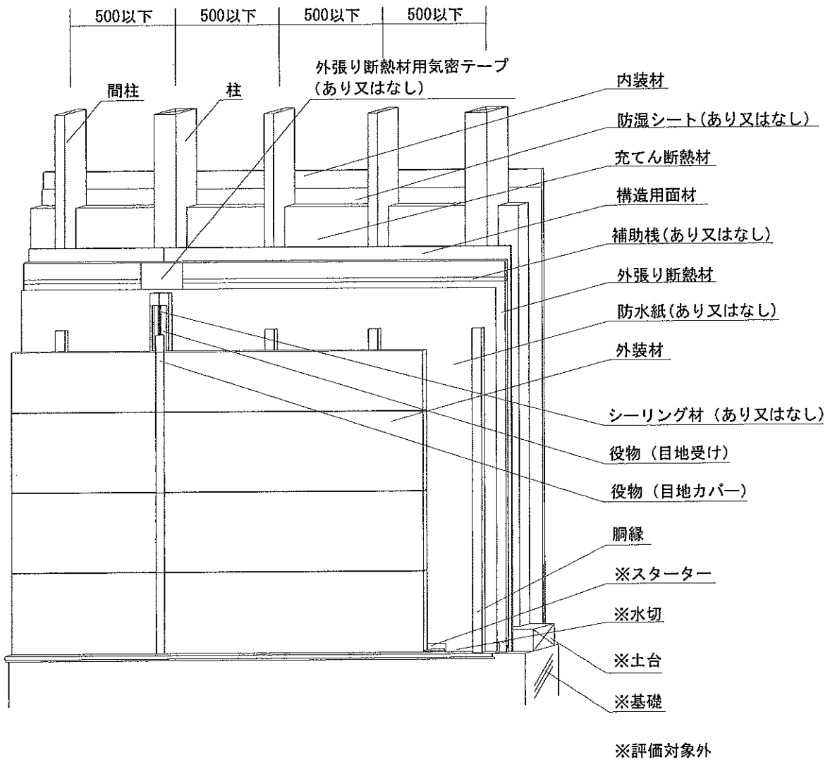
透視図
