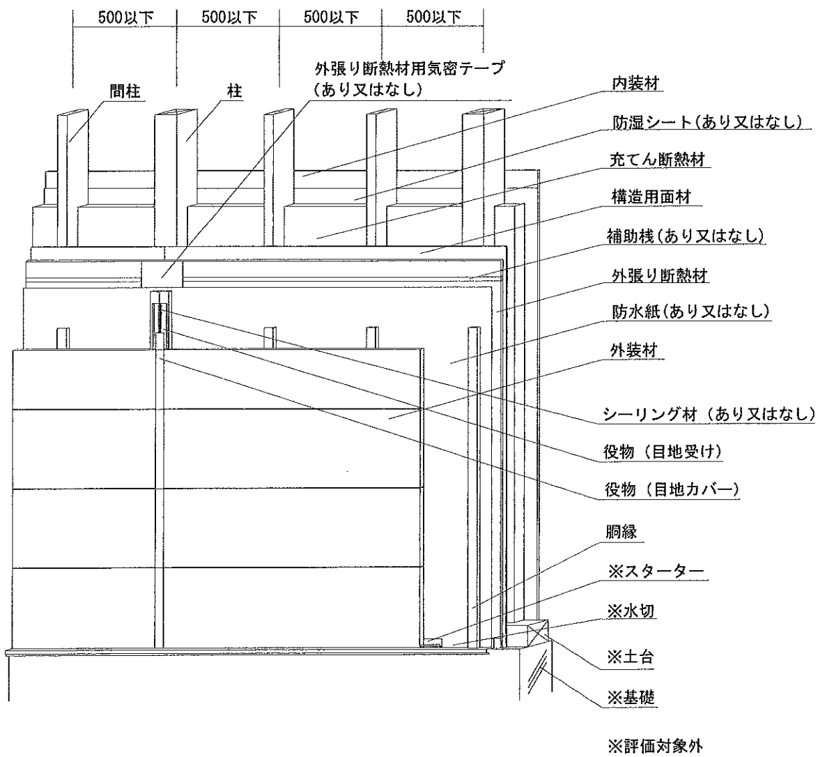
透視図
