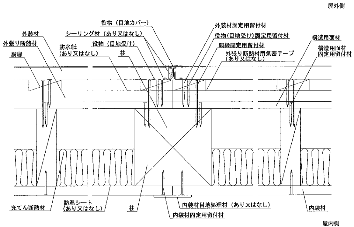
水平断面図
