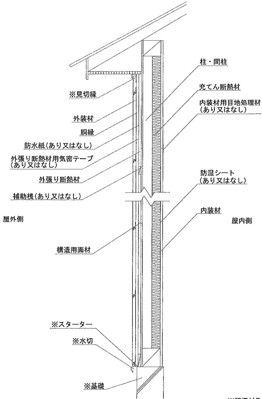
鉛直断面図
