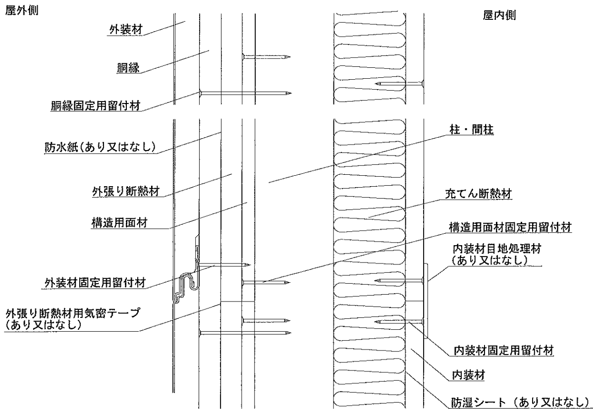
水平断面図
